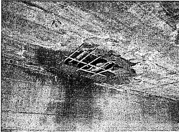
Estado puente k12+400 Losa
