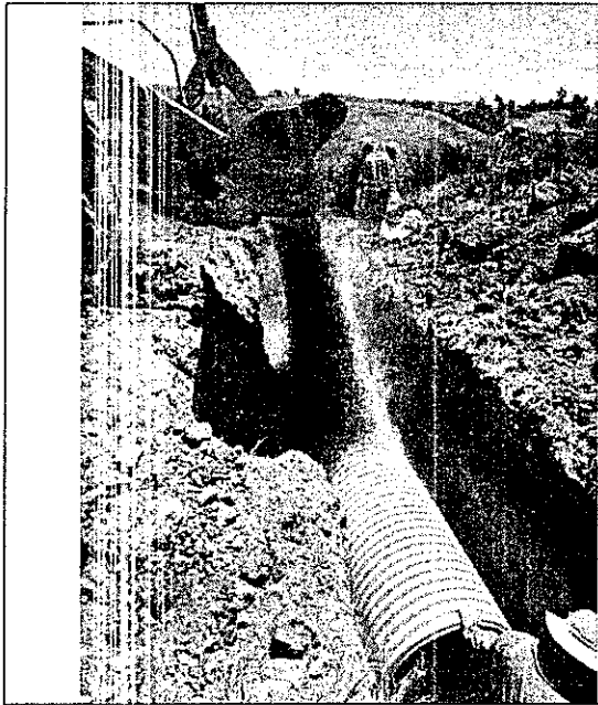
Construcción alcantarilla
