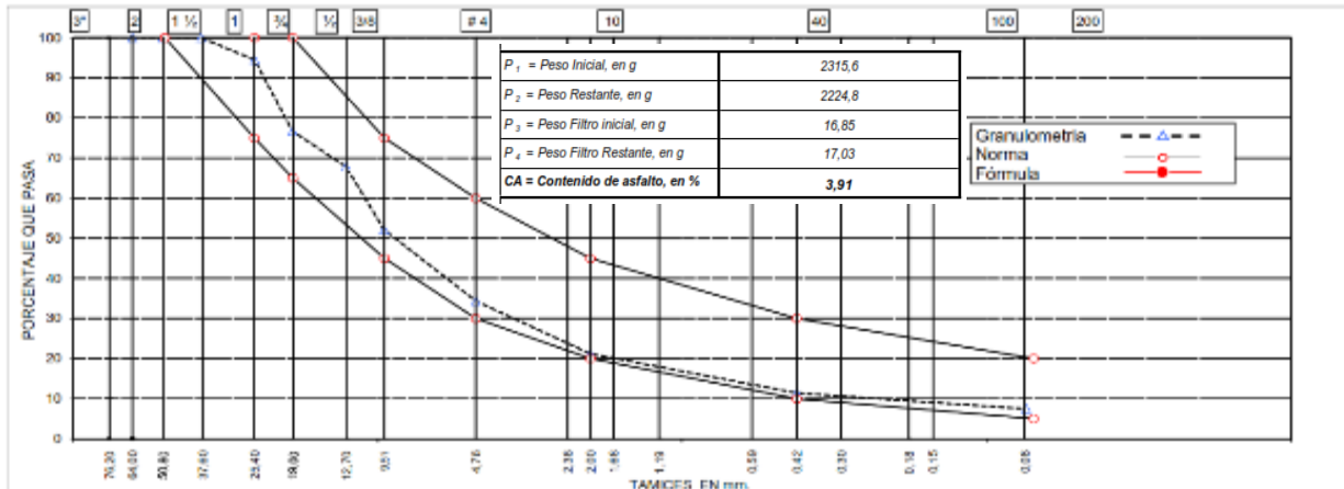
Grafica No. 1 – Caracterización Base estabilizada Km 12+300 Eje
