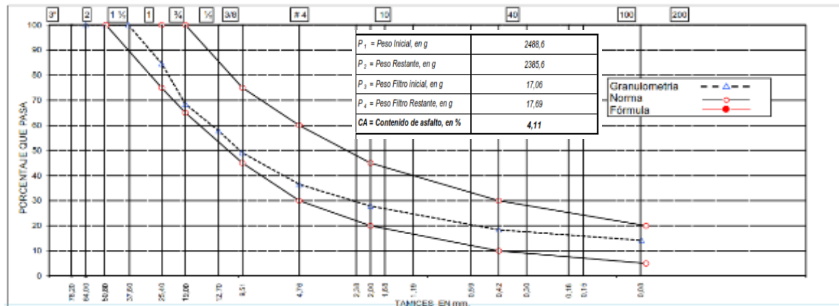
Grafica No. 2 – Caracterización Base estabilizada Km 1+350 Eje
