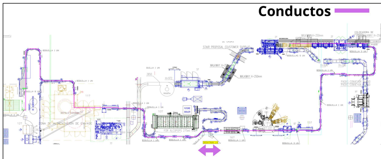
Ilustración 2 Ruta del sistema de Jabón lubricante y ubicación de boquillas L4
