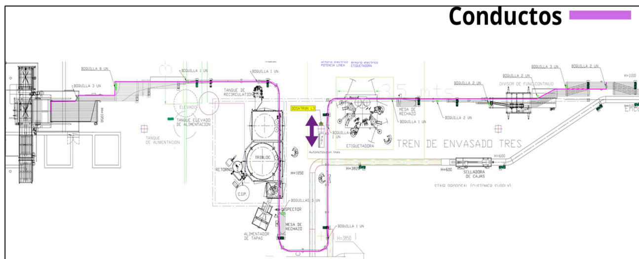
Ilustración 1 Ruta del sistema de Jabón lubricante y ubicación de boquillas L3
