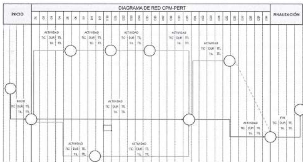
Esquema red, diagrama CPM/PERT, red medida
