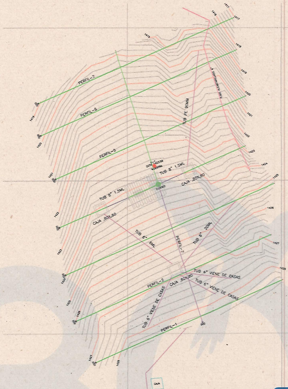
Imagen No.3. PTAR Manzanera No.2 Planta
