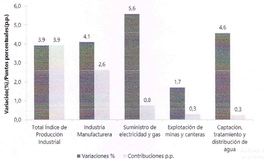
Gráfico 3. Variación y contribución anual del Índice de Producción Industrial por sectores industriales Total nacional Junio (2026 / 2025) Pr
