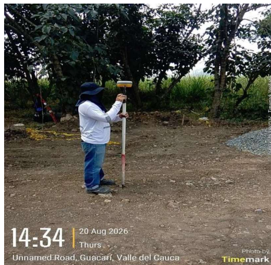
Ilustración 5. Referenciación instalación accesorios abscisa K4+560
