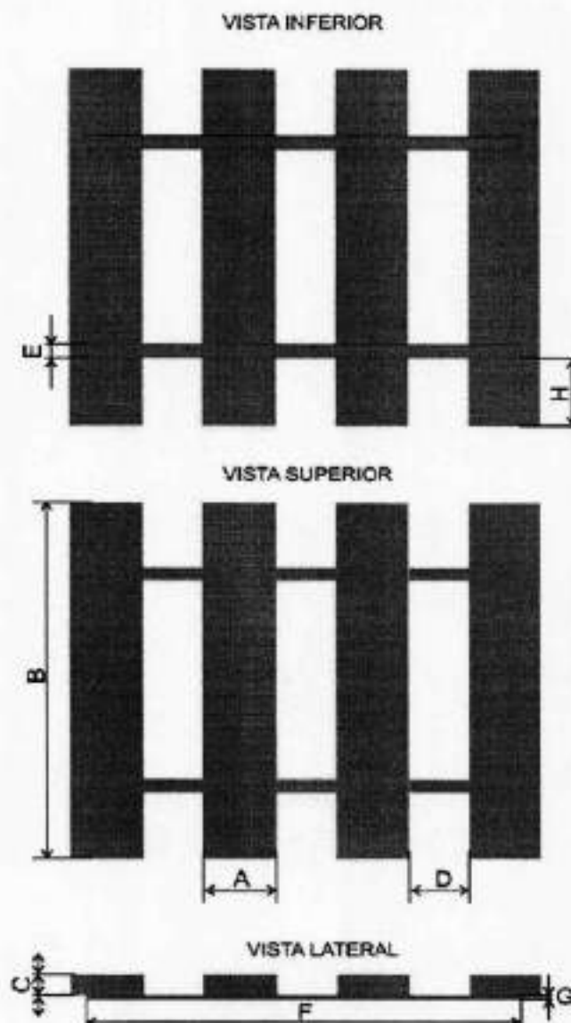
Figura 9. Tendido de madera
