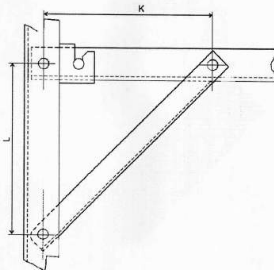
Figura 10. Detalle del refuerzo diagonal
