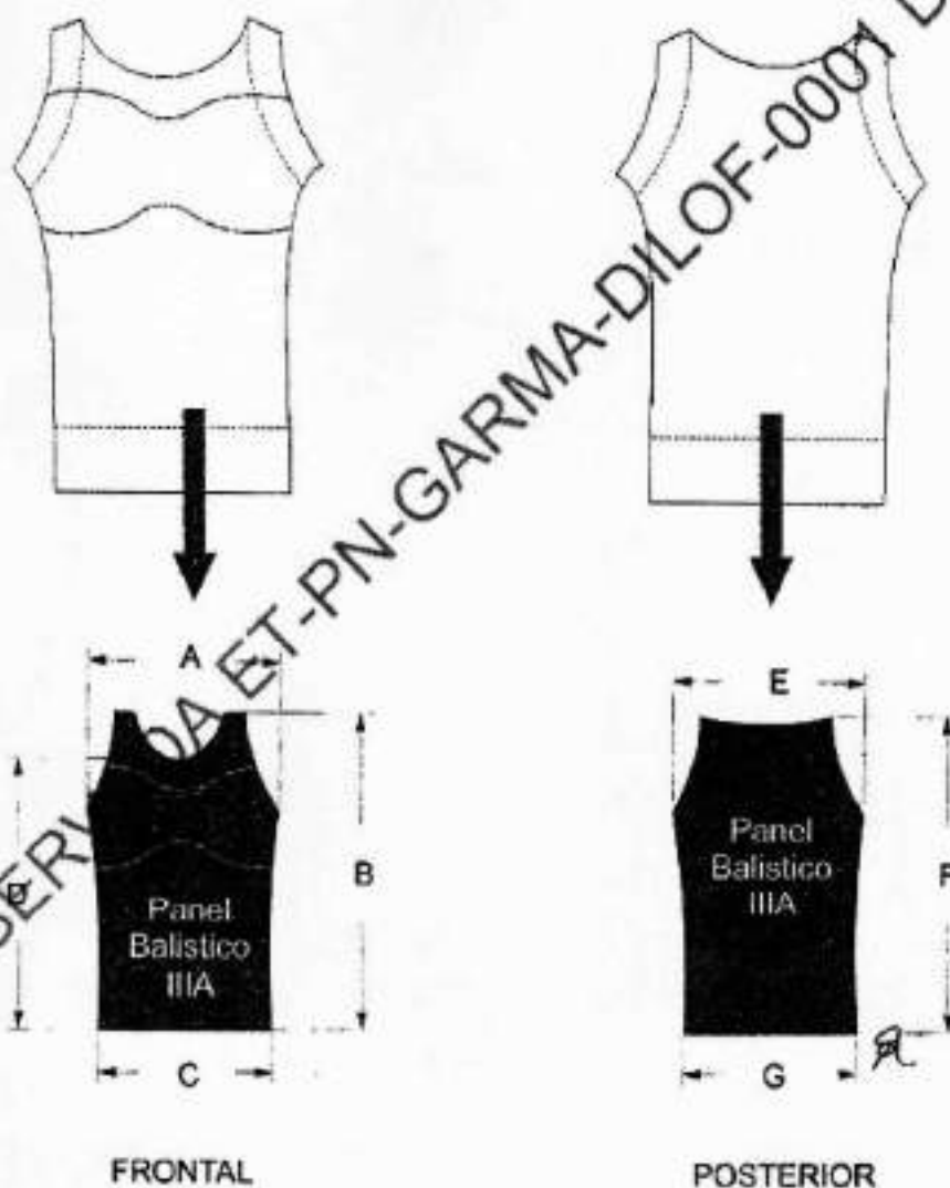
Figura 2. Diseño franela femenina
