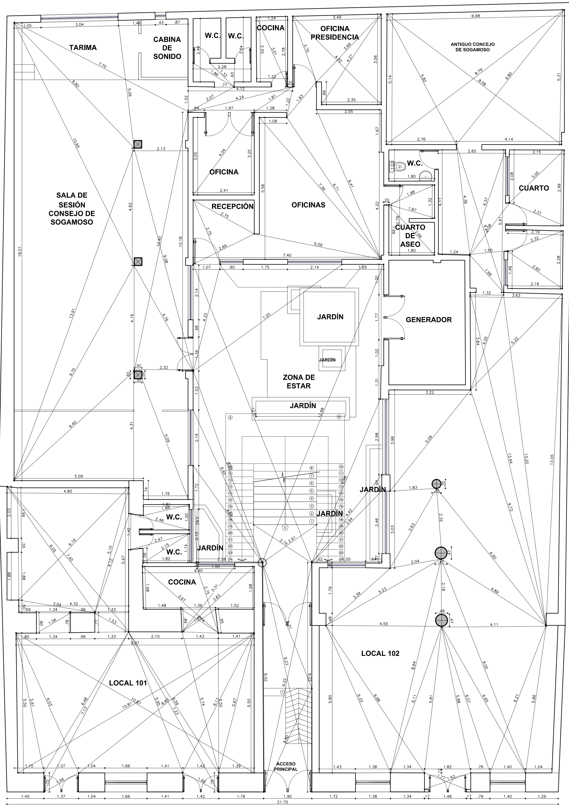
PLANTA PRIMER PISO ESC. 1:100
