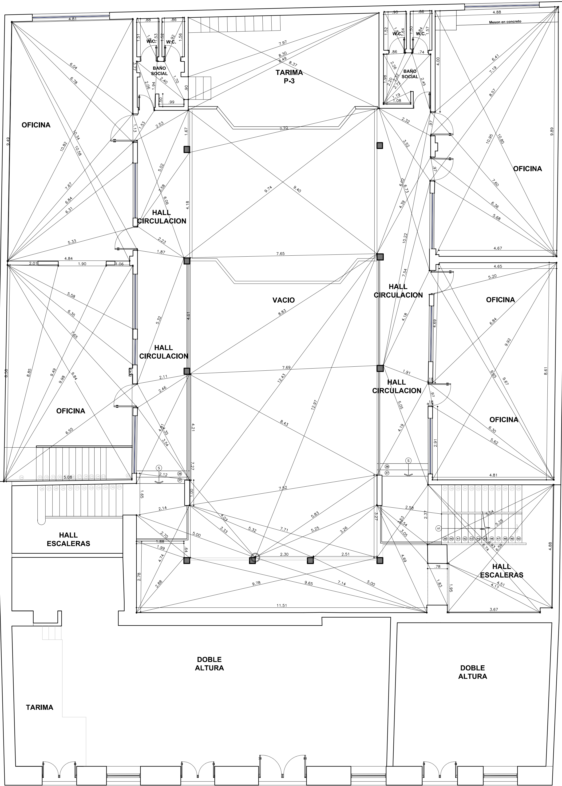
PLANTA TERCER PISO ESC. 1:100
