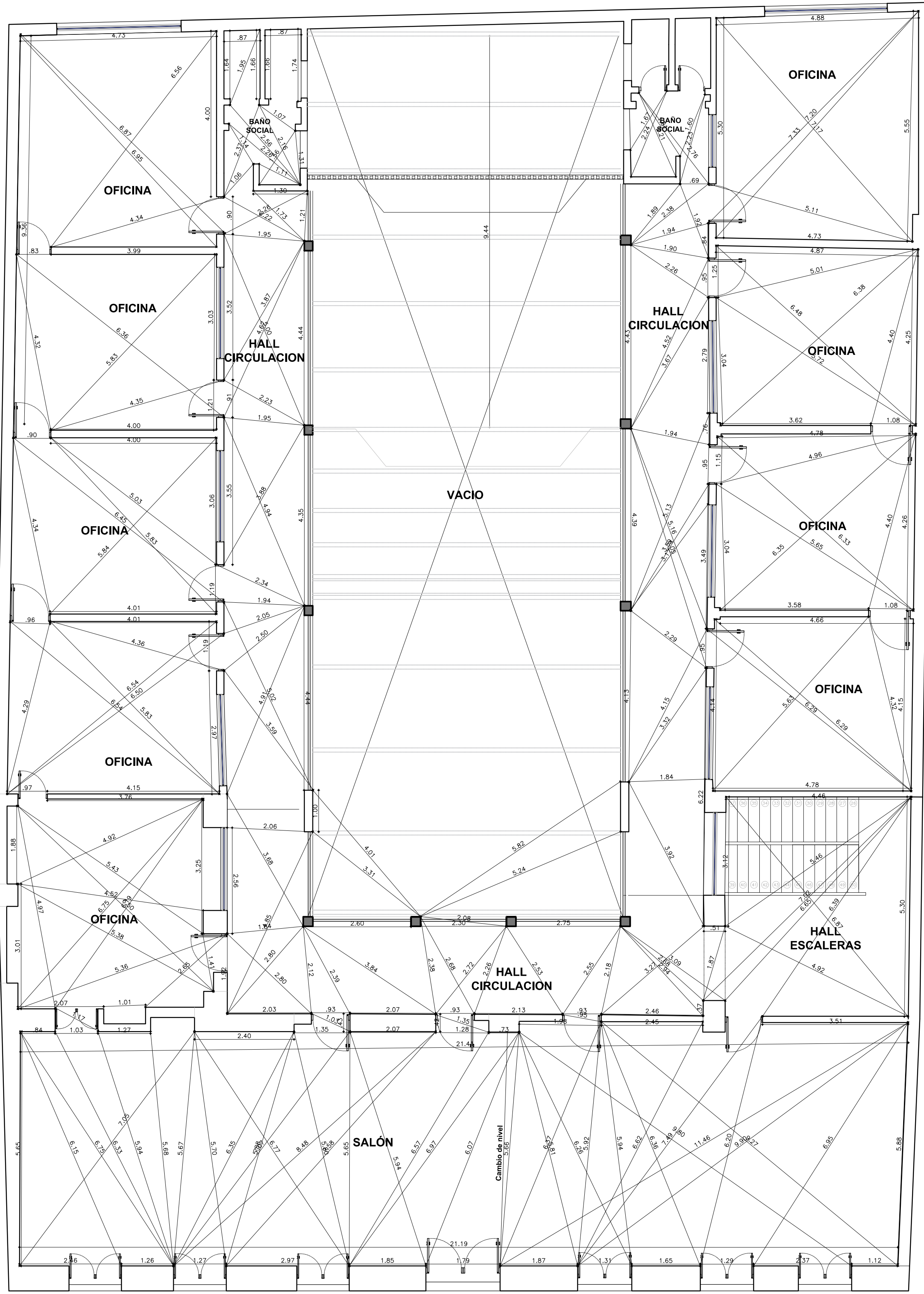
PLANTA CUARTO PISO ESC. 1:100
