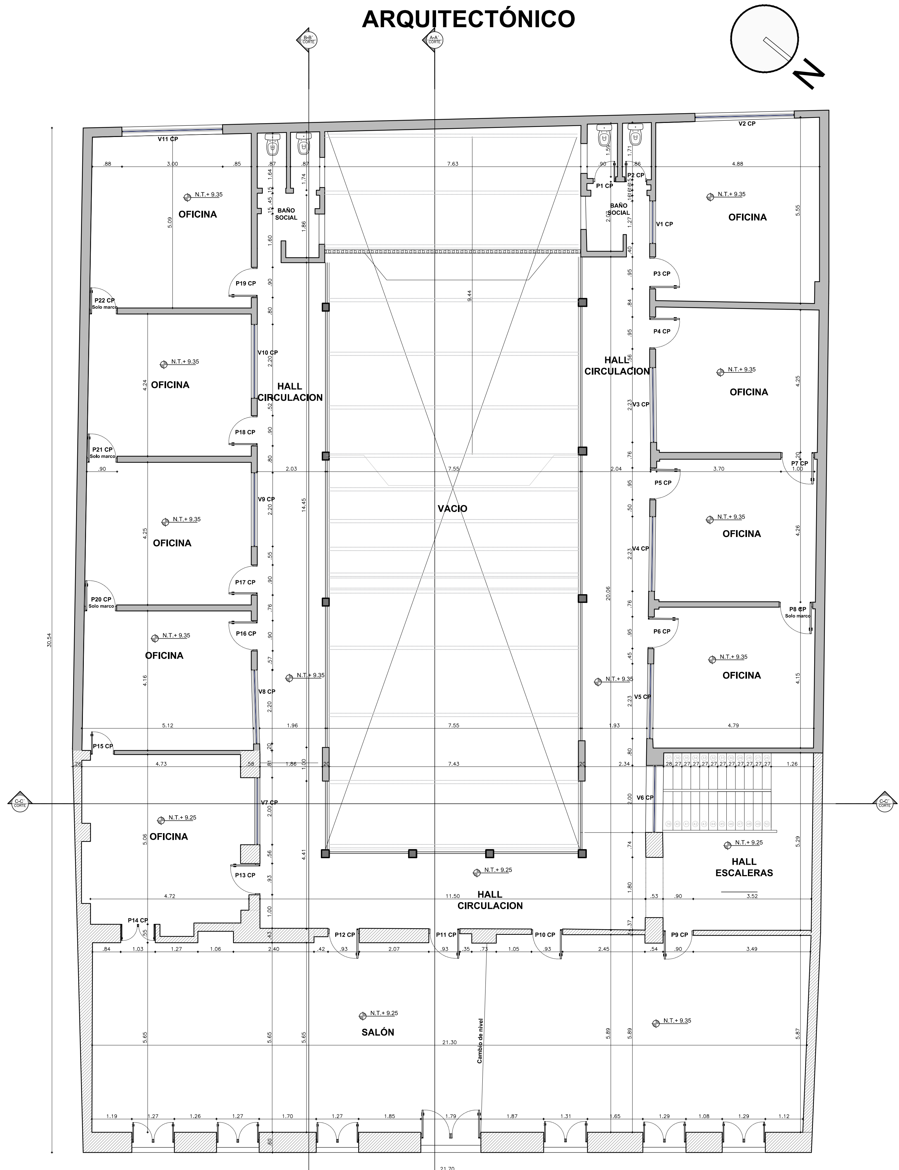
PLANTA CUARTO PISO ESC. 1:100
