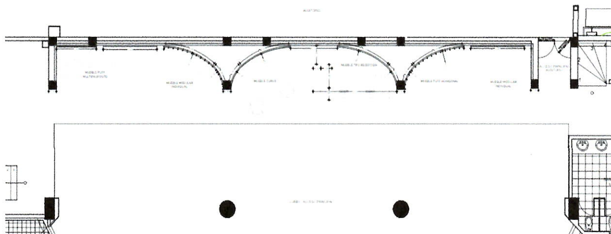
PLANTA ARQUITECTÓNICA
