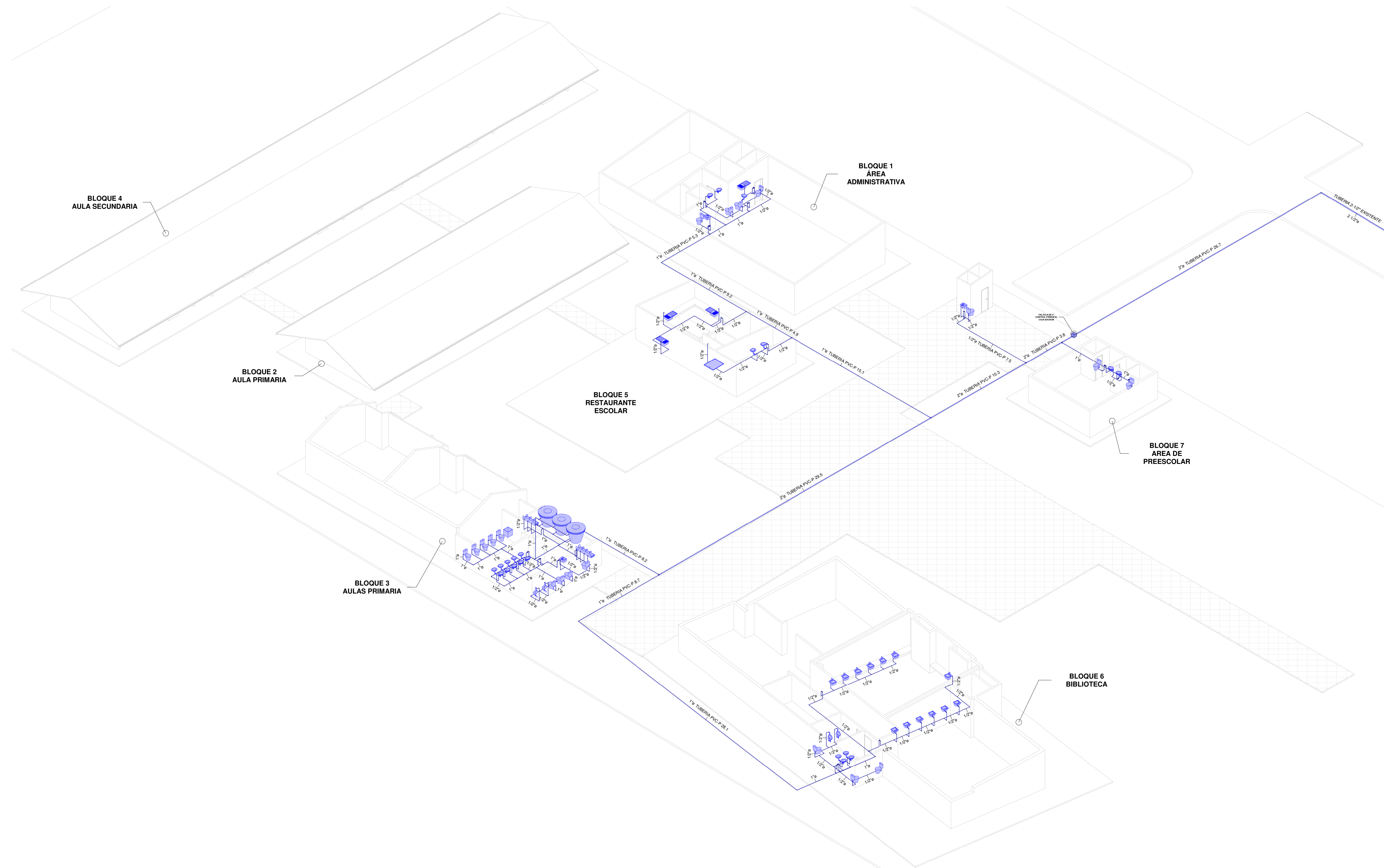
1 ISOMETRICO GENERAL-HID
