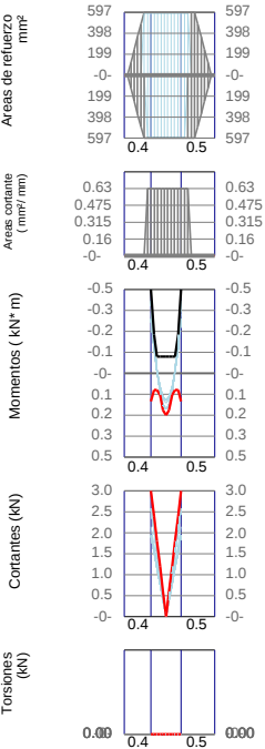
VCPrim13 / Base F'c=21\text{Mpa} Fy=420\text{Mpa} d'=60\text{mm}
