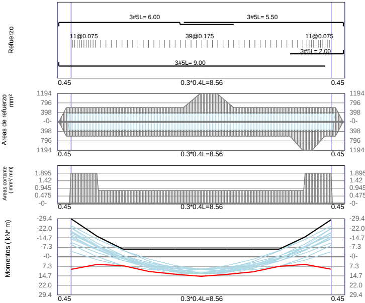
VPrim5 / Story2 F'c=21Mpa Fy=420Mpa d'=60mm
