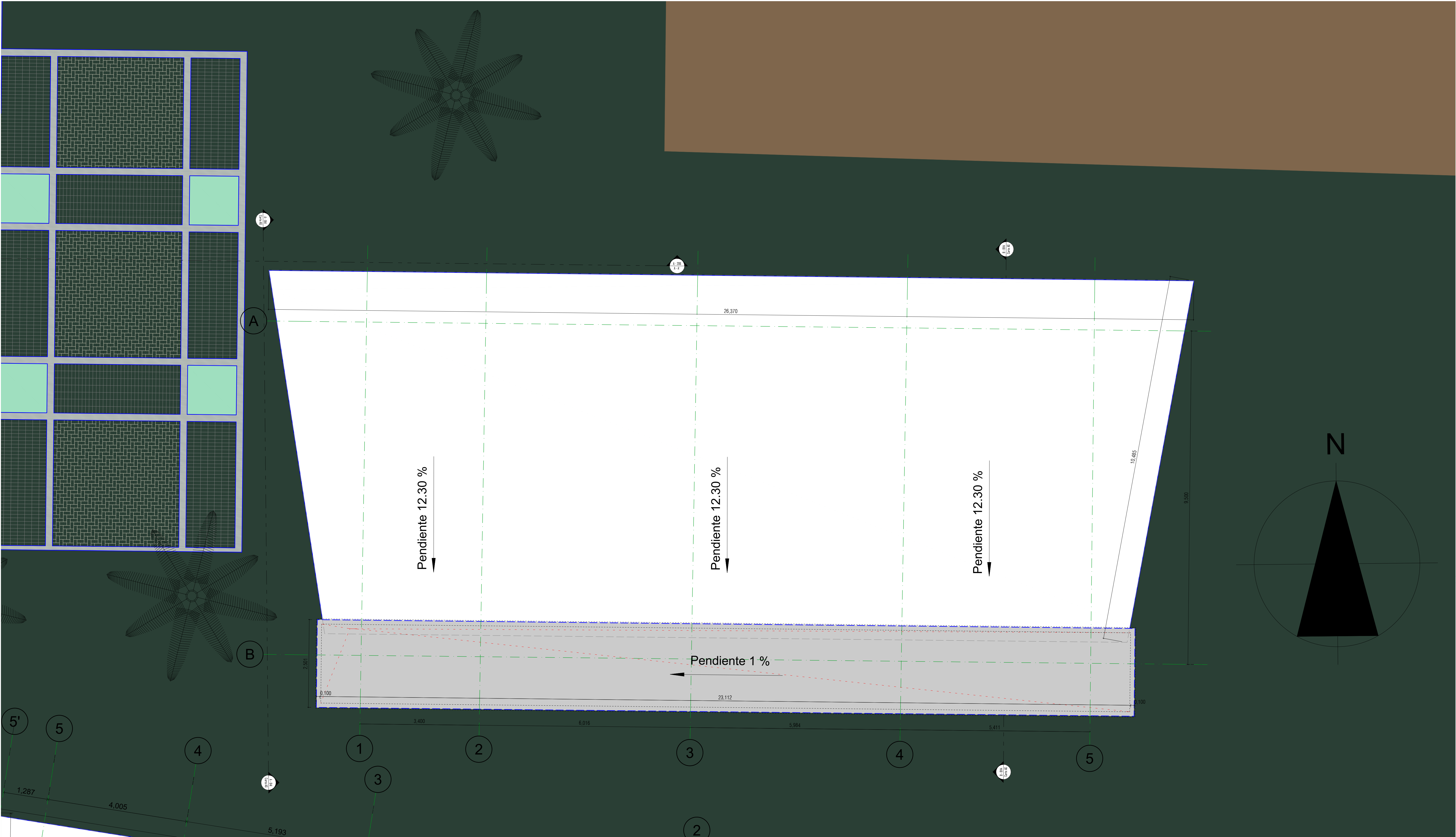
1 Planta Arquitectonica Bloque Administrativo 1:50
