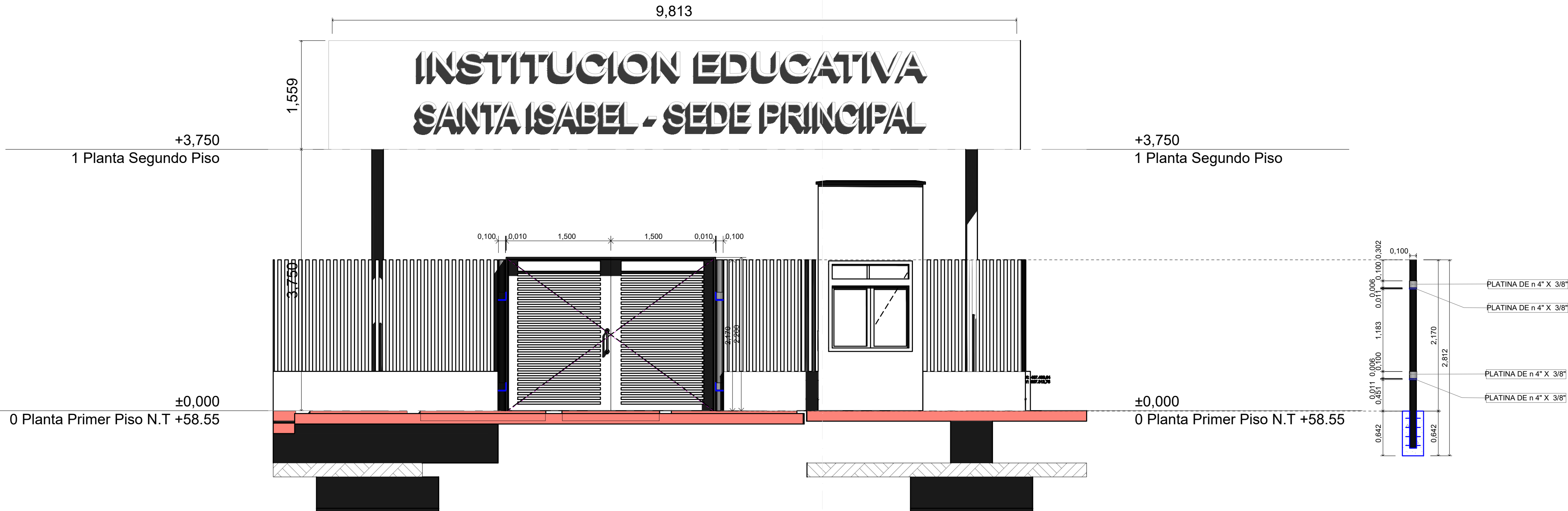
ESQUEMA SANTA ISABEL / CURUMANI 1:40,54
