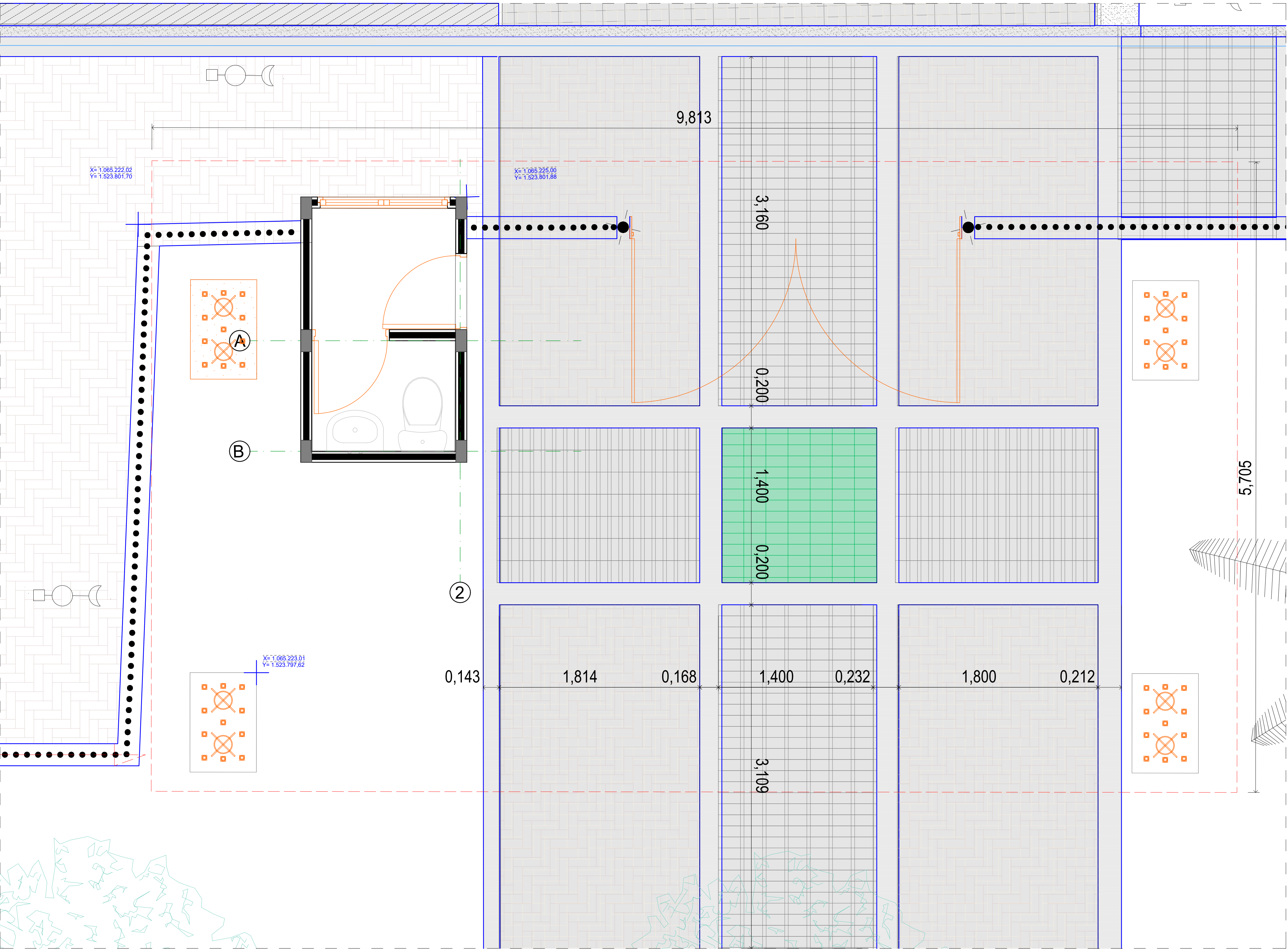
Detalle Pisos Plazoleta Acceso Principal 1:20
