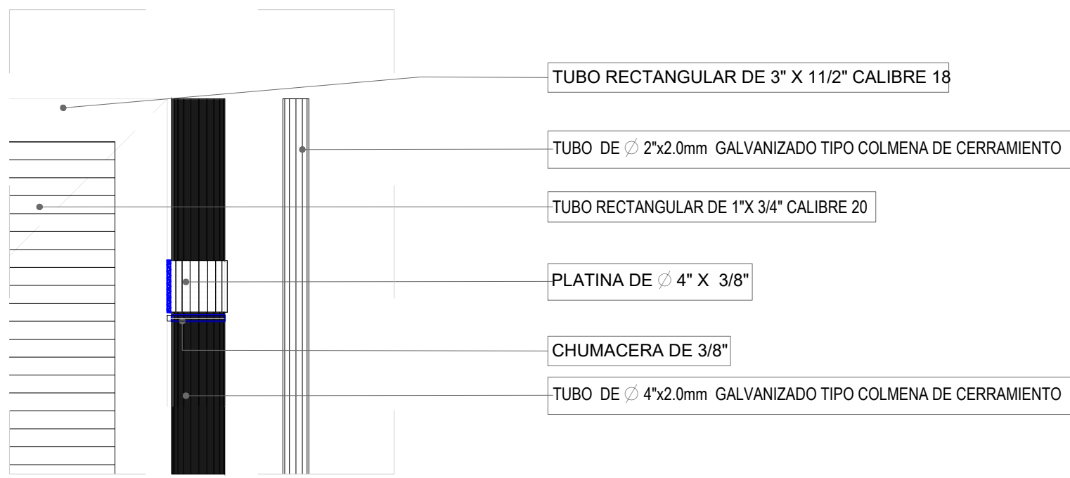
Detalle de Porton de Acceso 1:10
