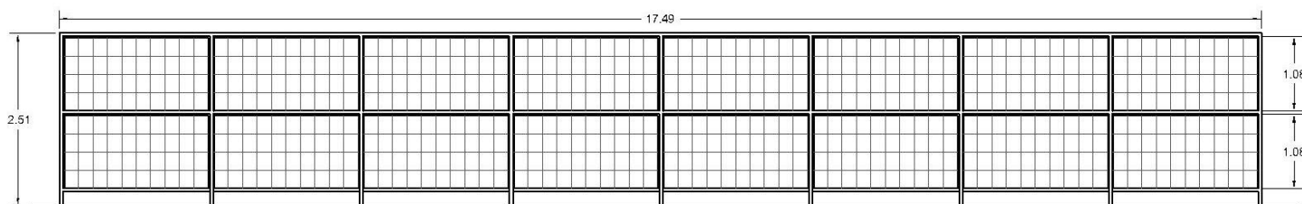
Alzado Estantería Altura Estándar Longitud larga (Nave Lateral). Cantidad: 2
