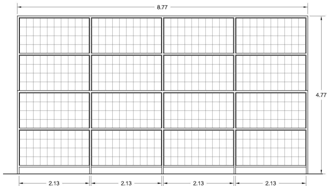
Alzado Estantería Doble Altura Longitud corta (Nave Central). Cantidad: 1
