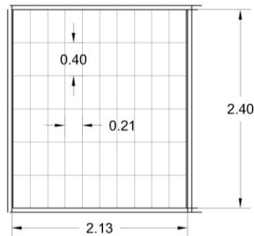
Detalle Distribución tipo de cajas Planta
