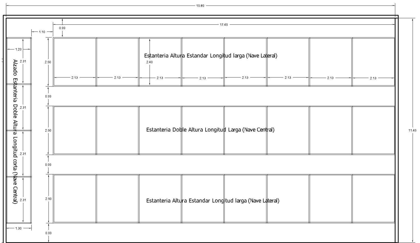
PLANTA DISTRIBUCIÓN DE ESTANTERIA
