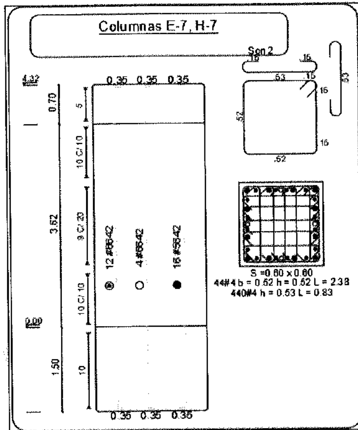
Nuevo despiece propuesto columnas E-7 y H-7
