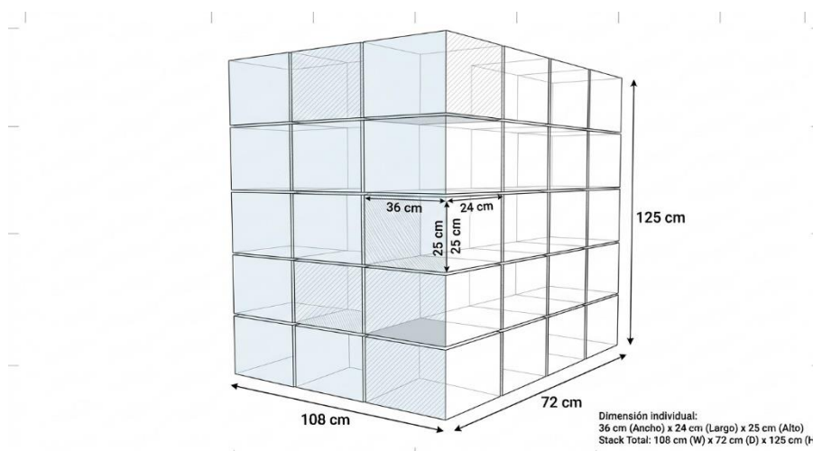
Gráfico 2. Pila de kits alimentarios.
