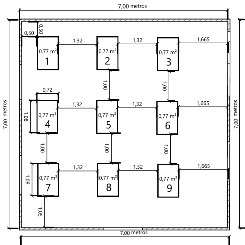
Gráfico 3. Vista superior 9 pilas de kits alimentarios en bodega de 7 x 7 metros.
