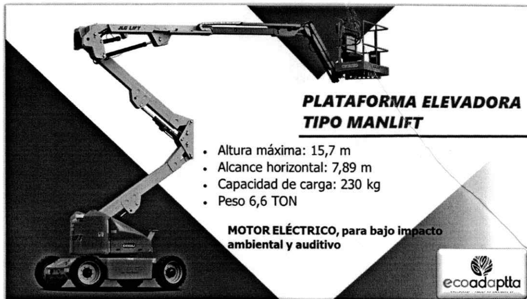
Plataforma elevadora tipo MANLIFT, propiedad de ECOADAPTTA
