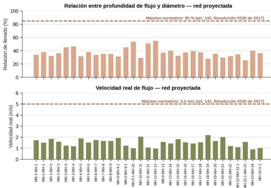
Gráfica 5. Verificación normativa de la red proyectada — relación de llenado y velocidad real
