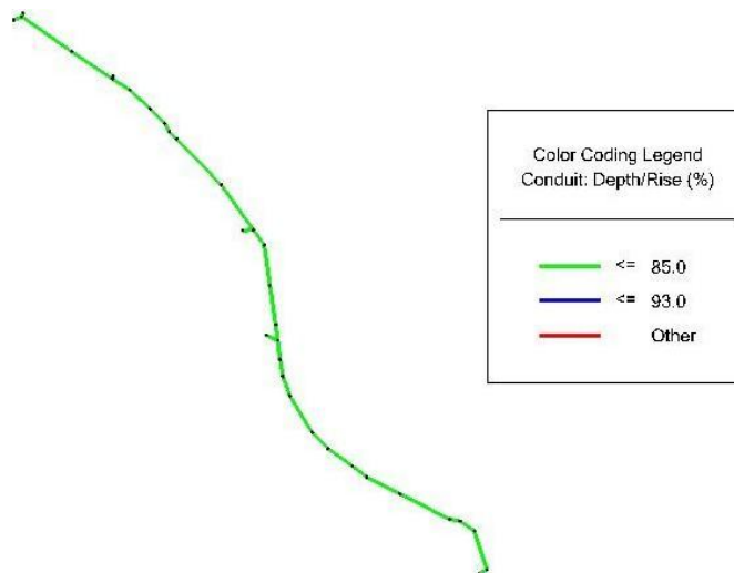
Ilustración 11. Evaluación de la relación de llenado — escenario de diseño
