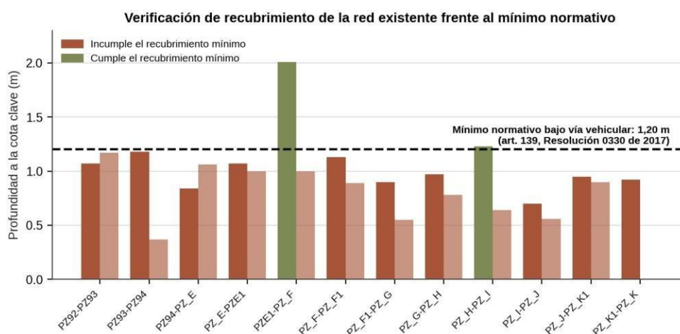
Gráfica 1. Déficit de recubrimiento de la red existente frente al mínimo normativo
