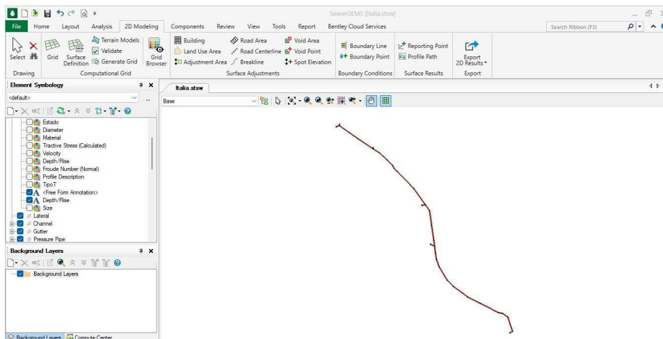
Ilustración 8. Topología de la red modelada en SewerGEMS
