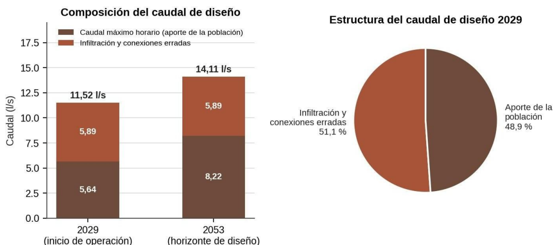
Gráfica 3. Composición y evolución del caudal de diseño del sector Italia 90
