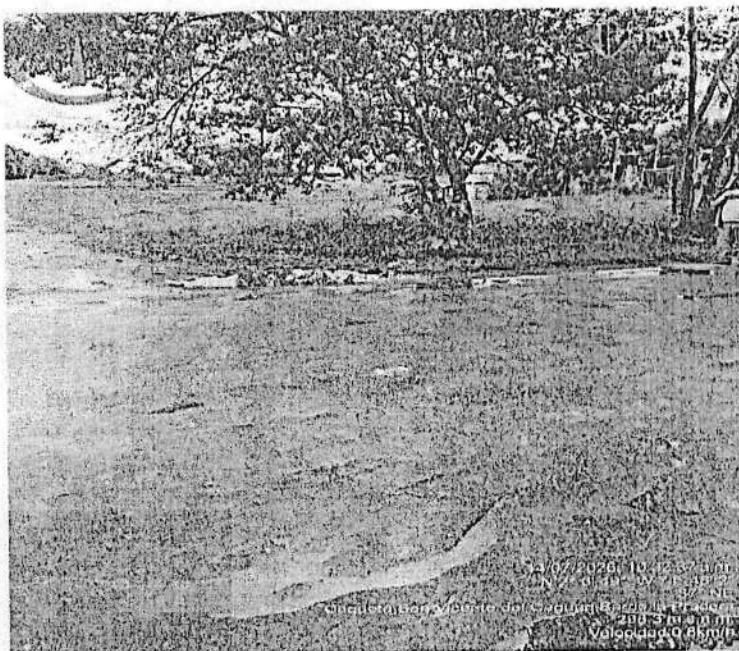
1 punto del cruce PR 49+957 escuela la arenoso, 6.90 mt ancho de vía- San Vicente Del Caguan
