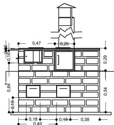
CORTE B-B
