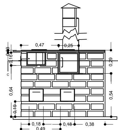
CORTE C-C
