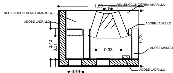
CORTE A-A
