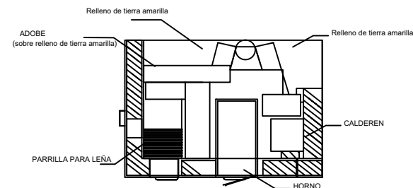
CORTE C-C
