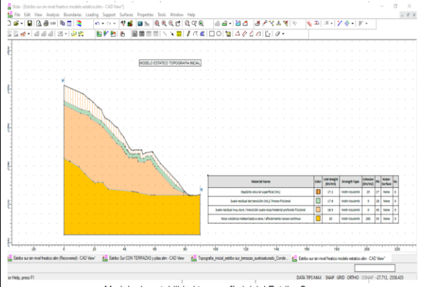
Imagen 4: Análisis Estabilidad de Taludes
