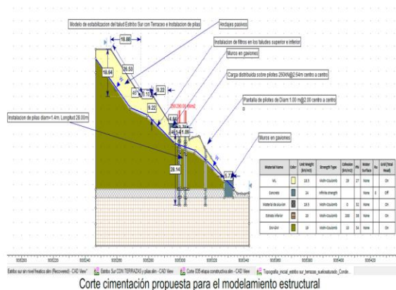
Imagen 3: Estabilización Sector Crítico
