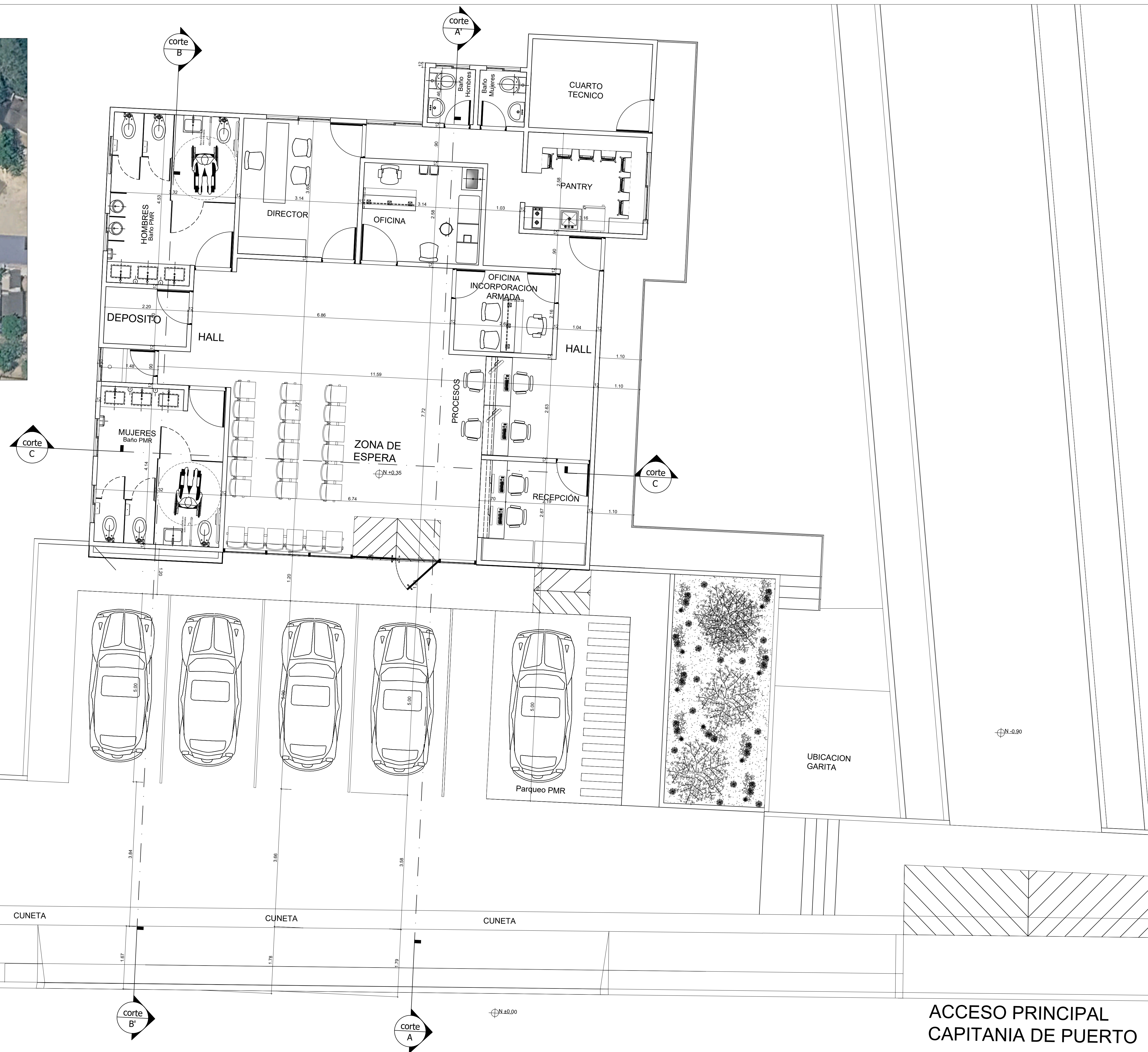
PLANTA PROPUESTA FRONT OFFICE COVEÑAS ESC 1:50
