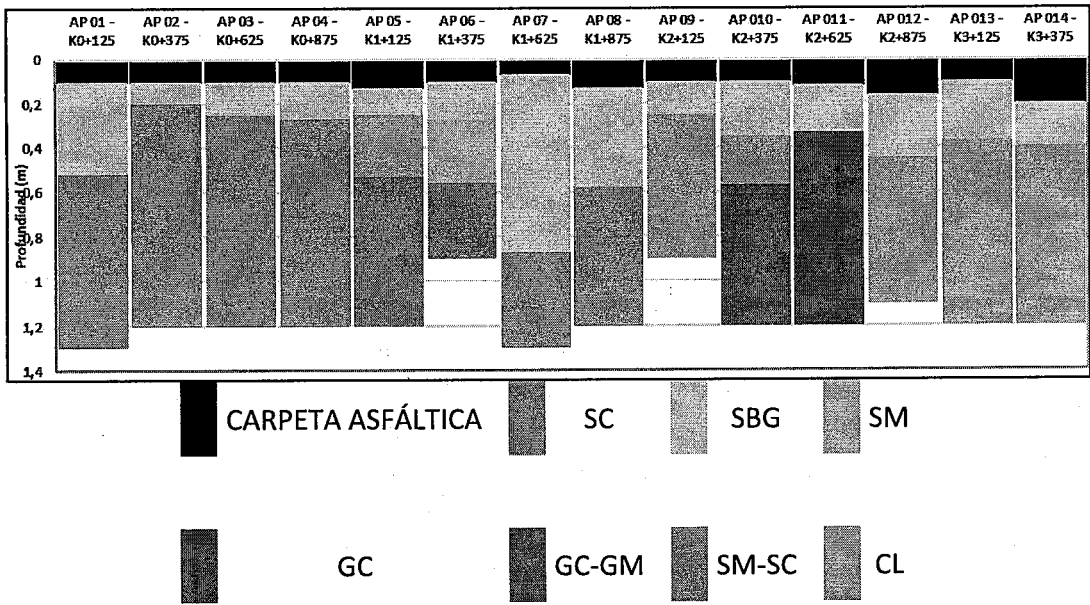
Figura 1. Modelo geológico – geotécnico. Fuente: Alcaldía de Fusagasugá, 2026.
