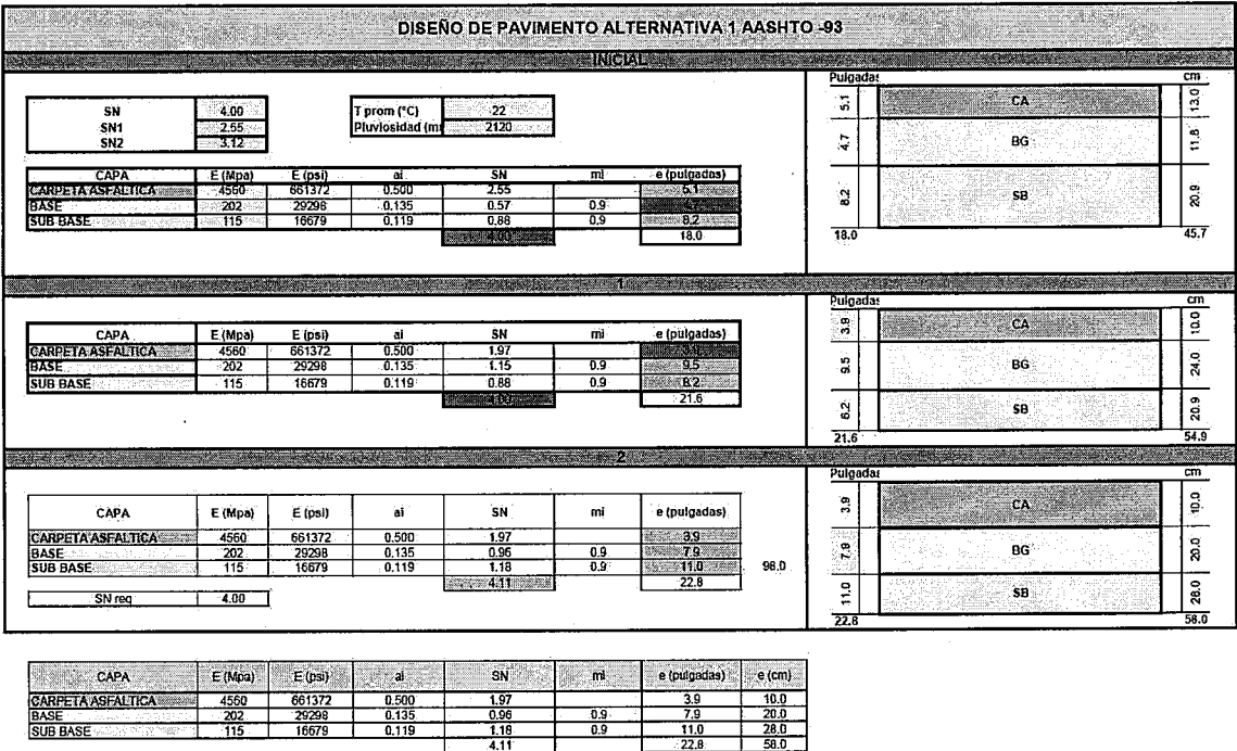
Figura 5. Cálculo de estructura de pavimento. Fuente: Alcaldía de Fusagasugá, 2026.
