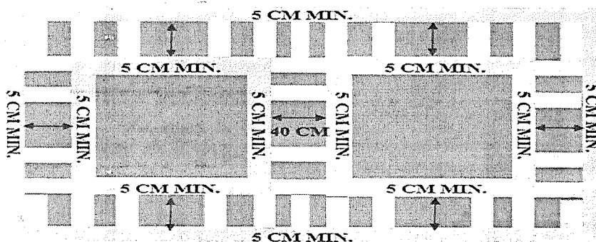
Imagen 1 (modelo de puestos de trabajo y libre circulación del técnico u operario (mecánico) con sus equipos y herramientas)
