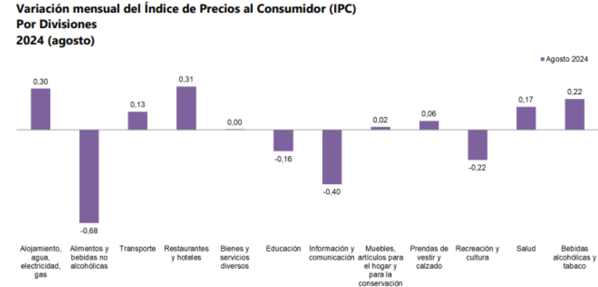
Gráfico 4. Variación y contribución mensual del IPC por divisionesde gasto
