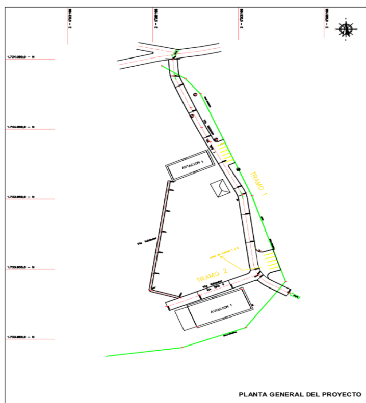
Figura 1.1. Planta general del proyecto BMMA1: Tramo 1 y Tramo 2.
