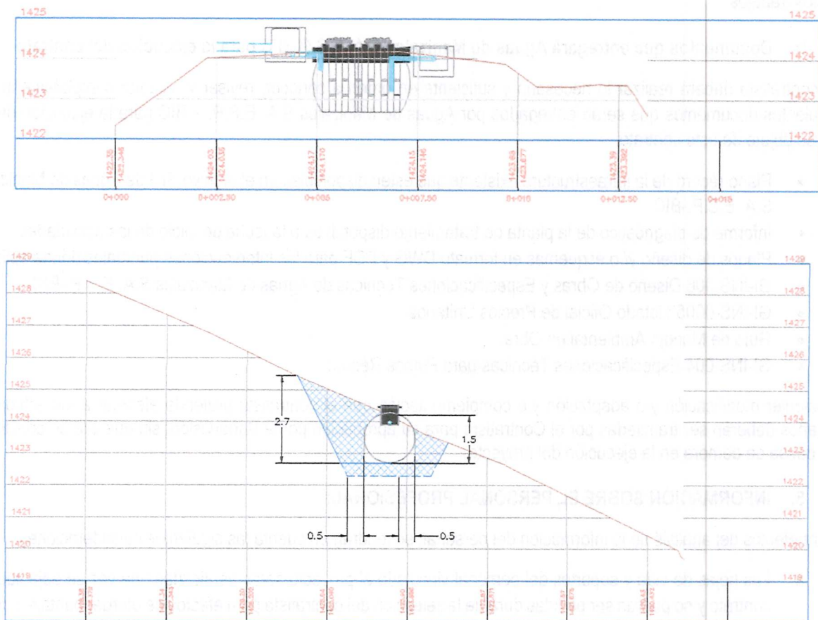
Imagen No.4. PTAR Manzanares No.2 Perfiles
