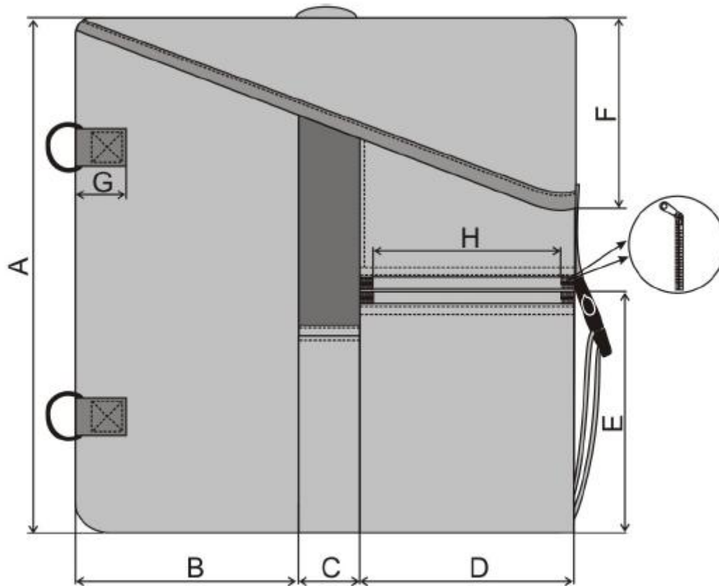
Figura 3. Vista lateral del morral
