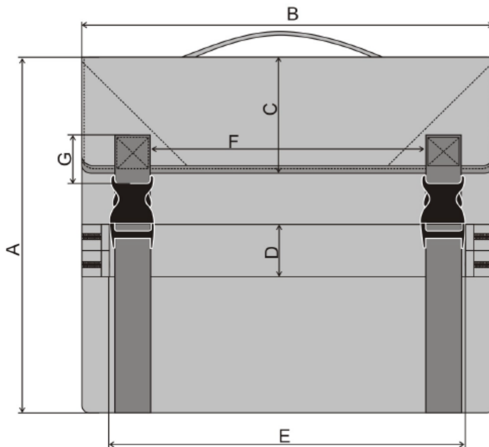
Figura 2. Vista frontal del morral
