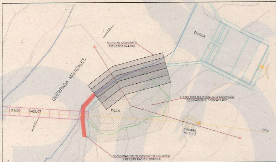
Imagen 2 – Obras de protección sector San Marcel Fuente – QUASAR Contrato 2025-0155
