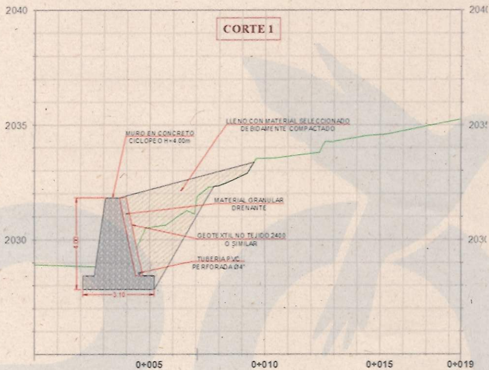
Imagen 7. Esquema de obras de protección San Marcel. Fuente – Quasar Contrato 2025-0155
