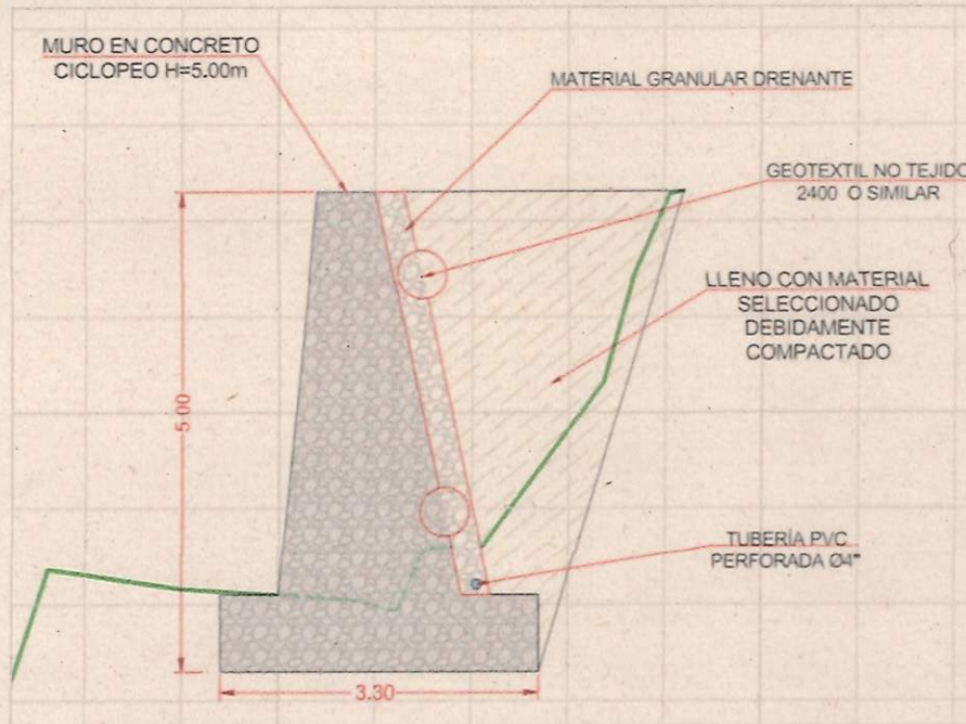
Imagen 6. Esquema de obras de protección Siselen. Fuente – Quasar Contrato 2025-0155
