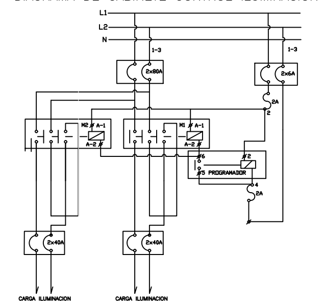
DIAGRAMA DE GABINETE CONTROL ILUMINACION
