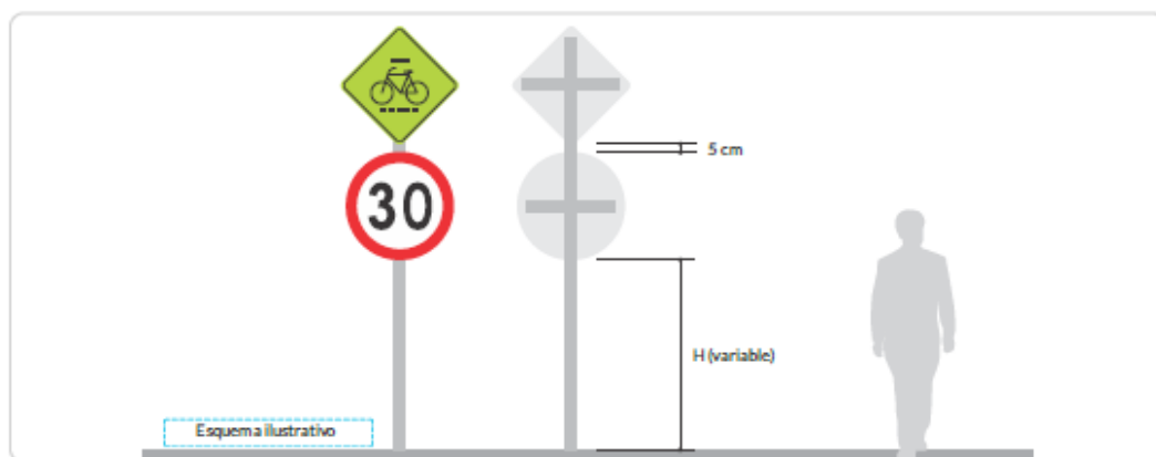
Figura 5: Ejemplo de la construcción de las señales dobles (DÚPLEX)
