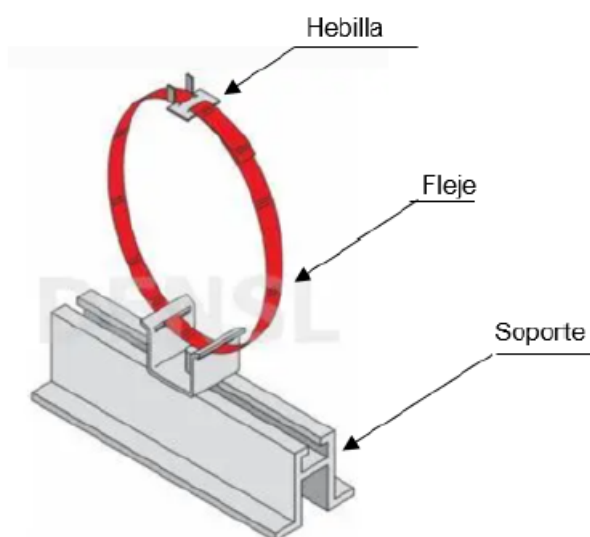
Figura 7: Sistema de sujeción mediante zunchado
