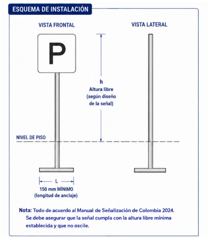
Figura 1: Instalación Señales Verticales.
