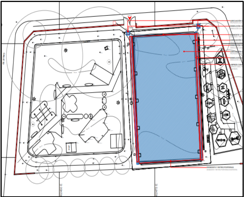
GRÁFICA 17: Planta General de implantación escenario La Independencia.
