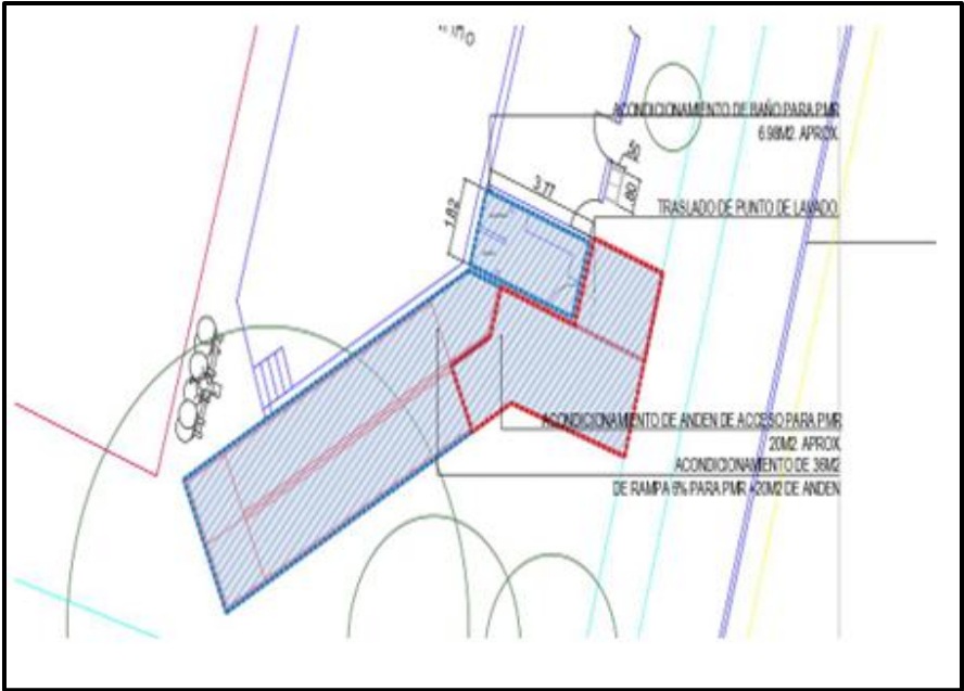
GRÁFICA 16: Planta General de implantación escenario deportivo el Guabal.
