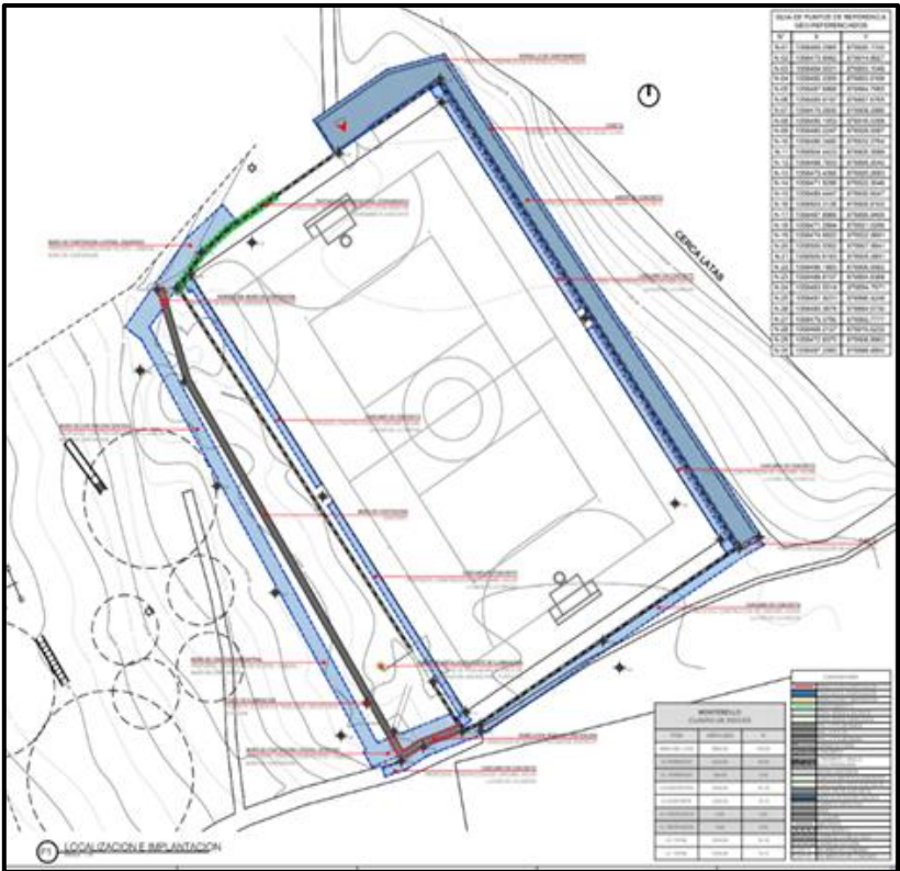
GRÁFICA 15: Planta General de implantación escenario cancha múltiple Montebello.
