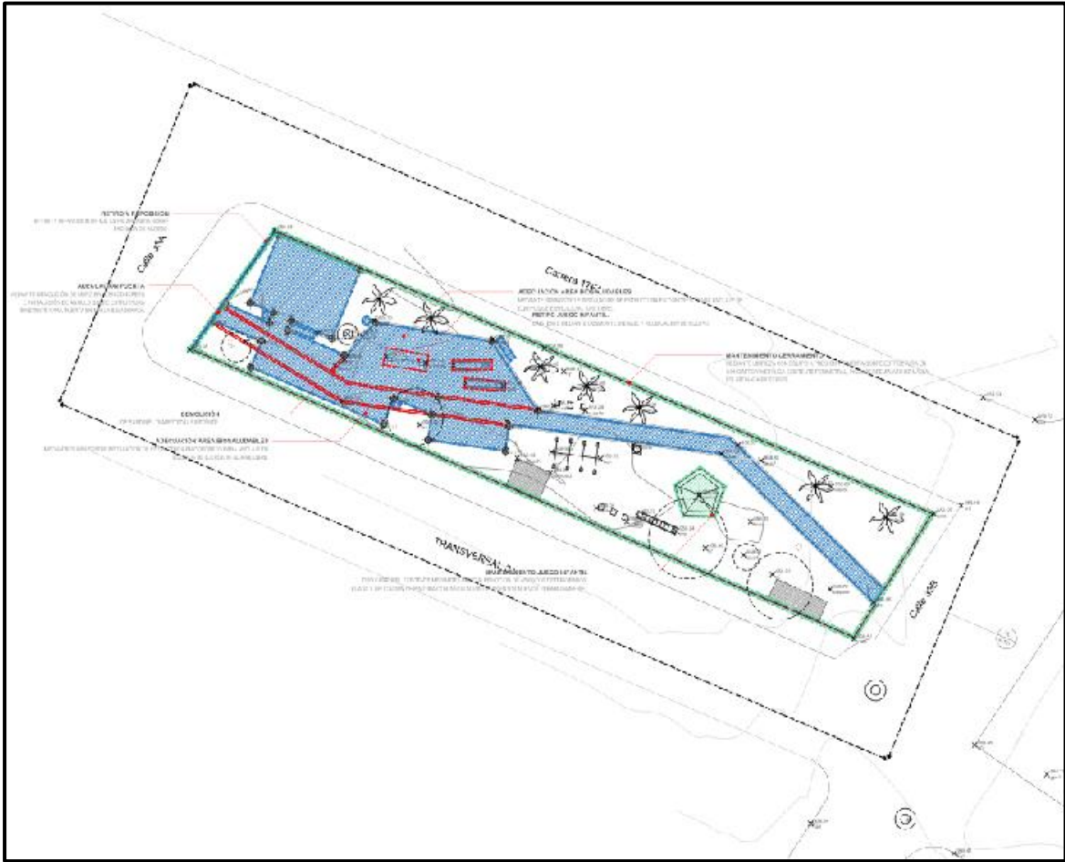
GRÁFICA 20: Planta General de implantación escenario deportivo Parque Recreativo y Deportivo Saavedra Galindo - Los Gatos.
