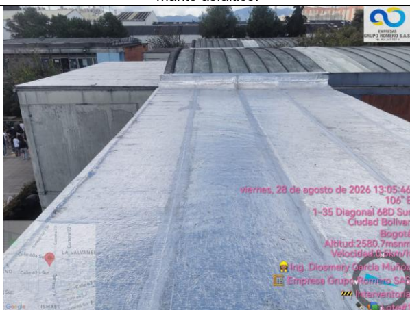
Se terminan actividades en bloque morado de instalación de manto asfáltico.
