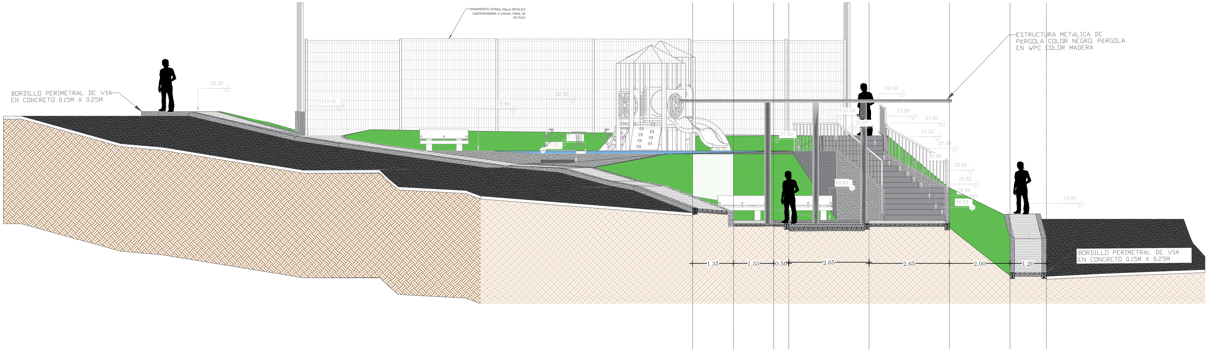
CORTE TRANSVERSAL 1
