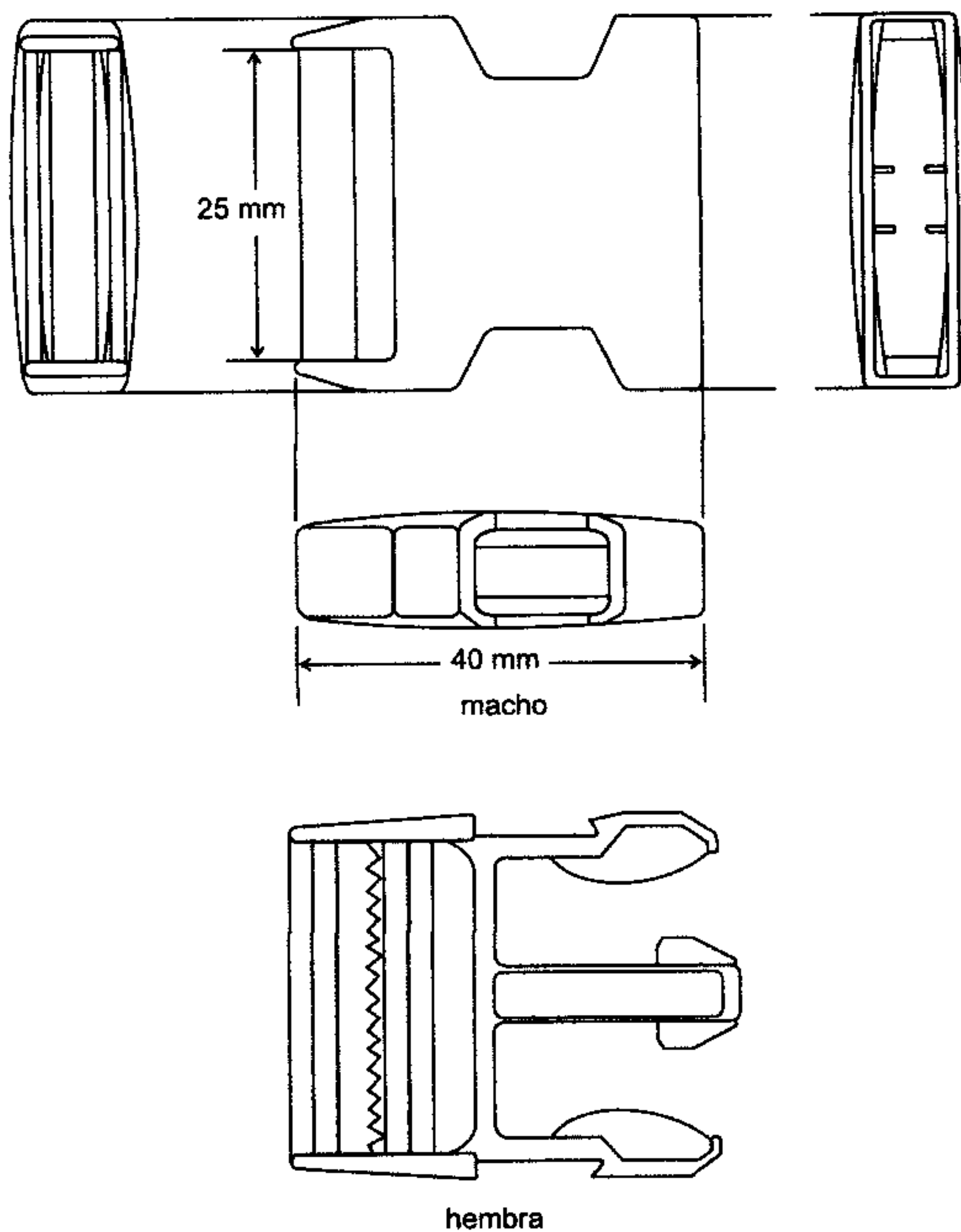
Figura 7. Modelo opcional, a manera de ejemplo chapa plástica suelta rápido - reata de 25 mm
