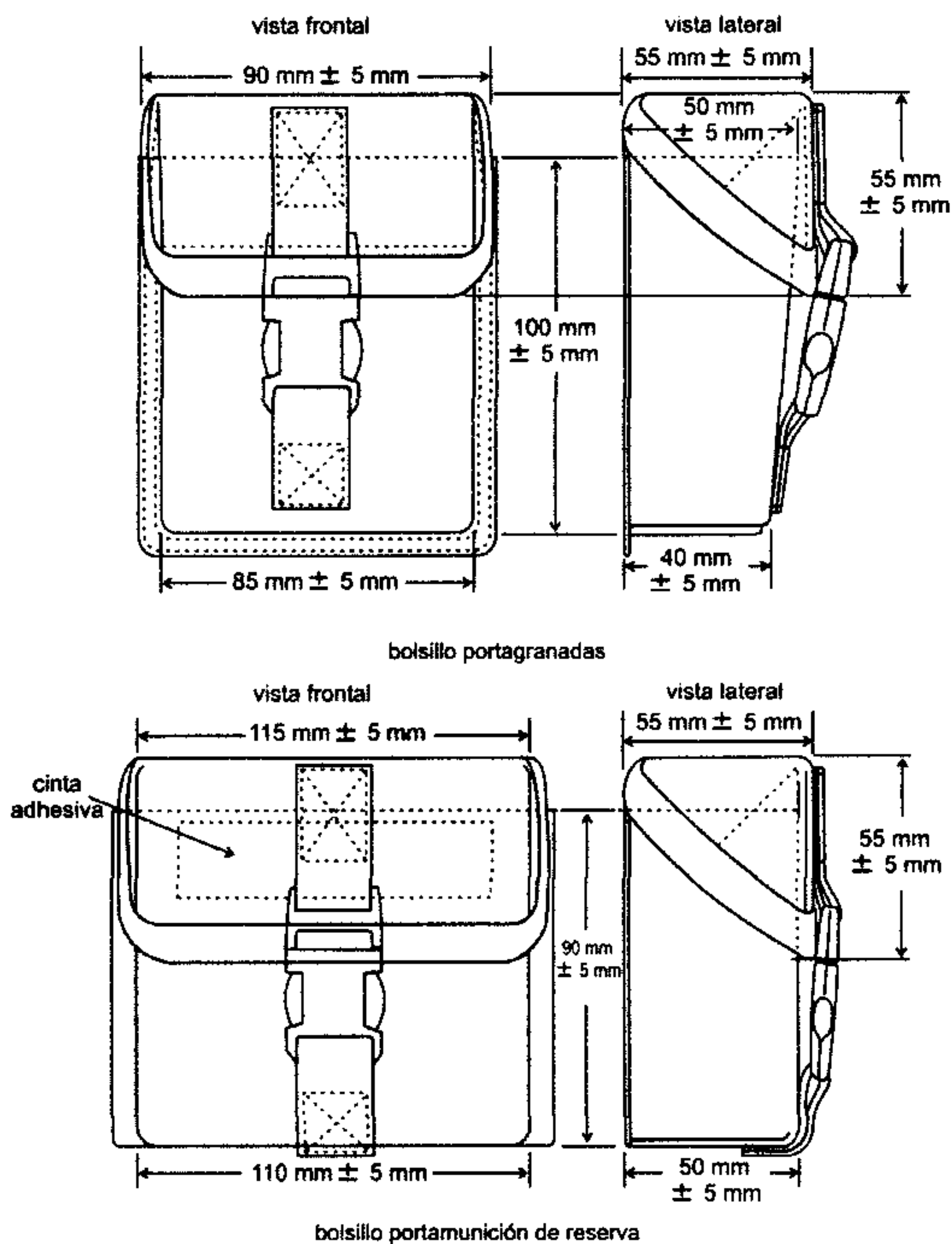
Figura 8. Bolsillo portagranadas y bolsillo potamunición
