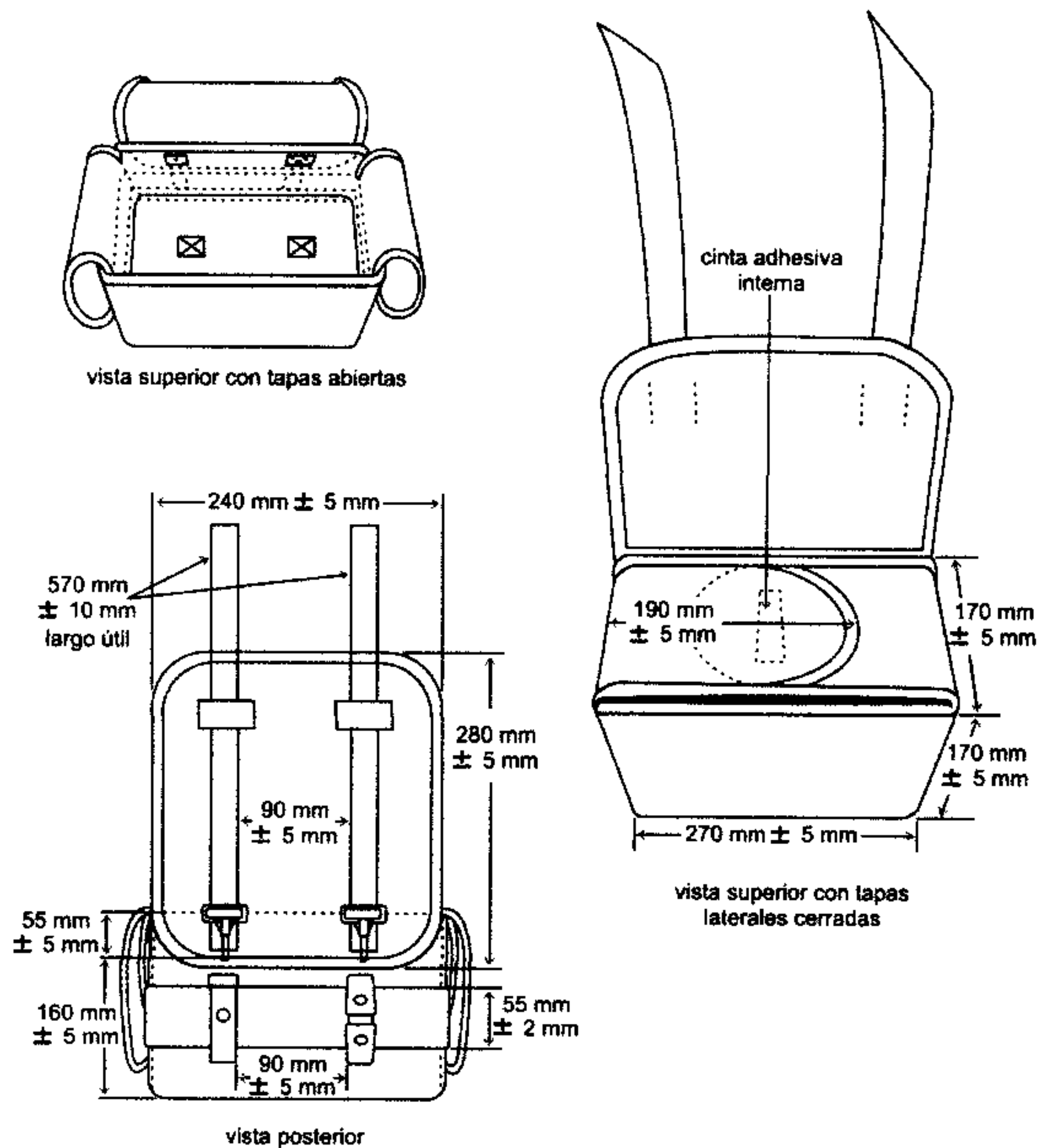
Figura 5. Bolso multiusos (vistas diferentes)
