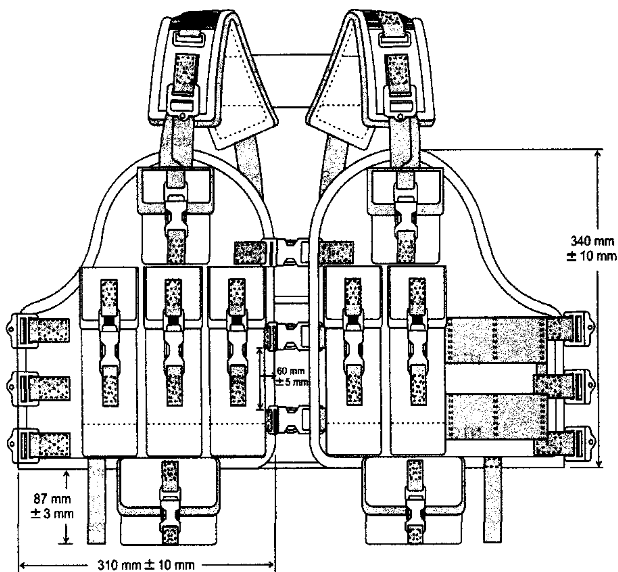
Figura 1. Confección chaleco diez proveedores vista frontal
