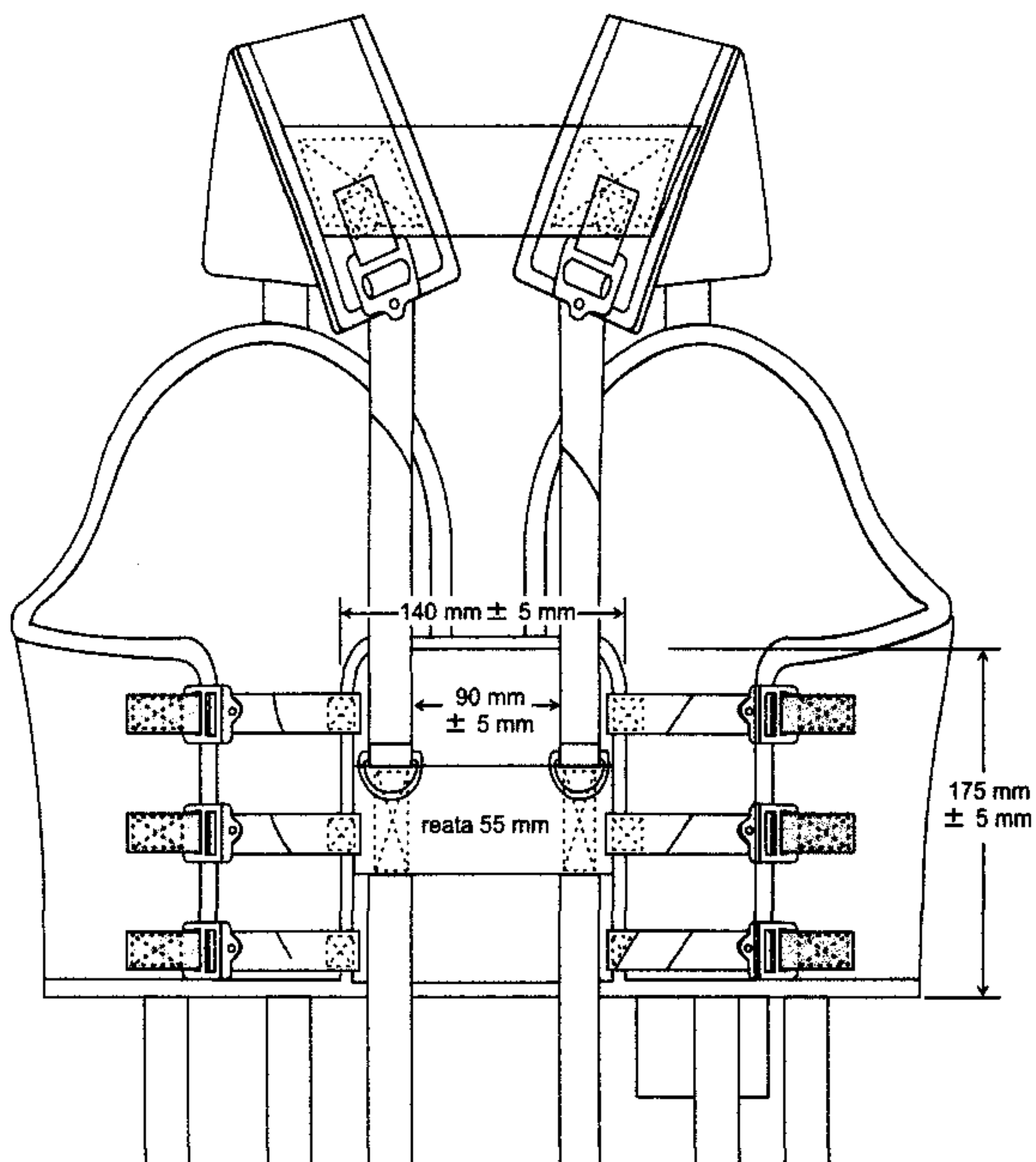
Figura 3. Confección chaleco diez proveedores vista posterior
