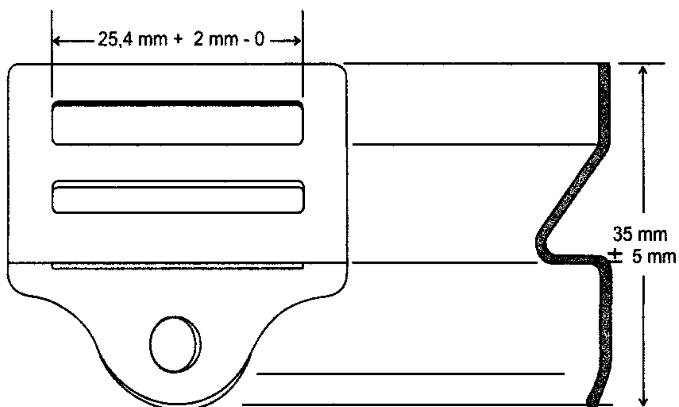
Figura 9. Hebilla doble puente de 25 mm (prototipo)
