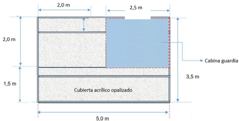
IMAGEN 3. VISTA SUPERIOR DE LA ESTRUCTURA
