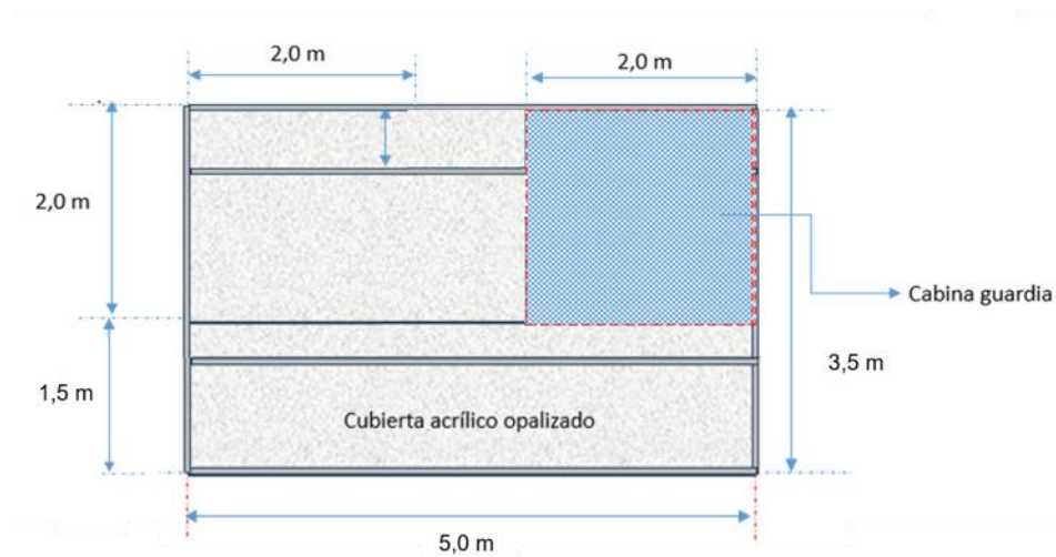
IMAGEN 3. VISTA SUPERIOR DE LA ESTRUCTURA
