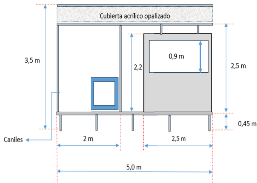
IMAGEN 1. VISTA FRONTAL DE LA ESTRUCTURA
