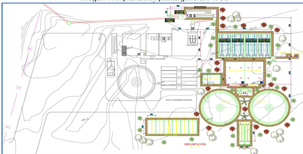
Imagen 1. Implantación planta general PTAR.
