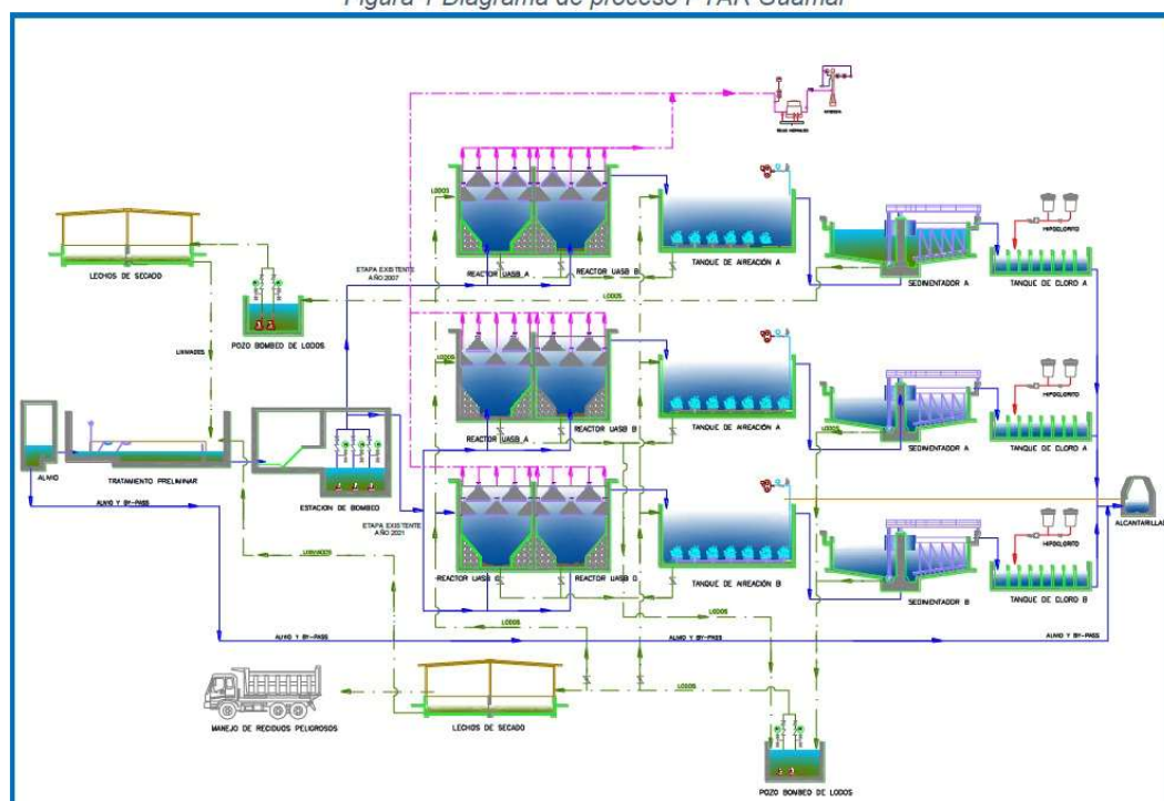
Figura 1 Diagrama de proceso PTAR Guamal
