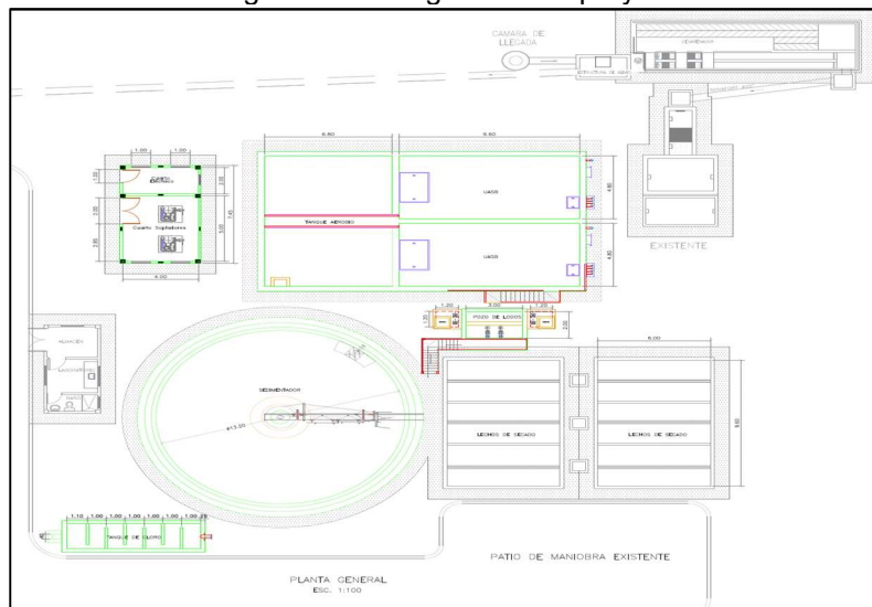
Imagen 2. Planta general del proyecto.
