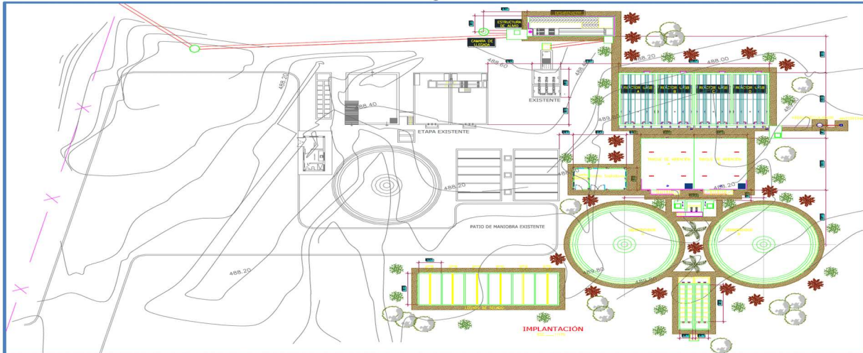
Imagen 1. Implantación planta general PTAR.
