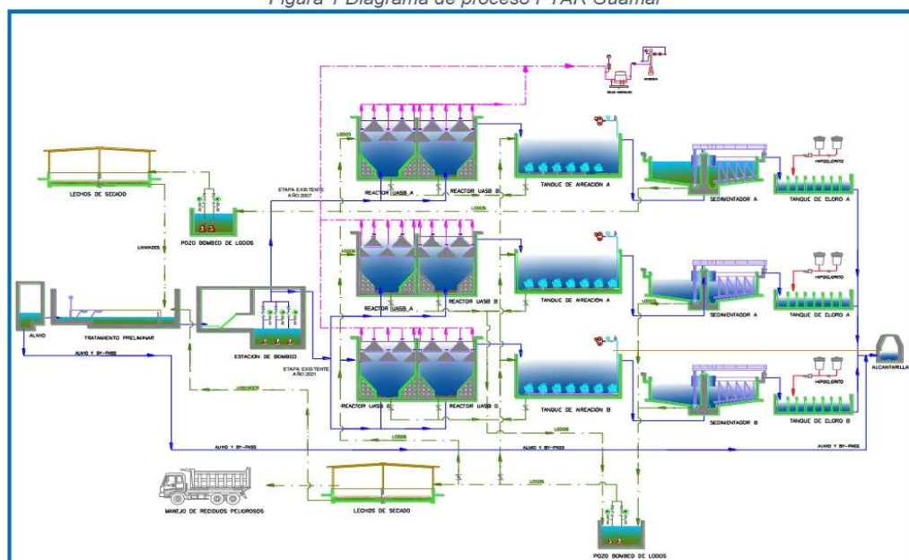
Figura 1 Diagrama de proceso PTAR Guamal
