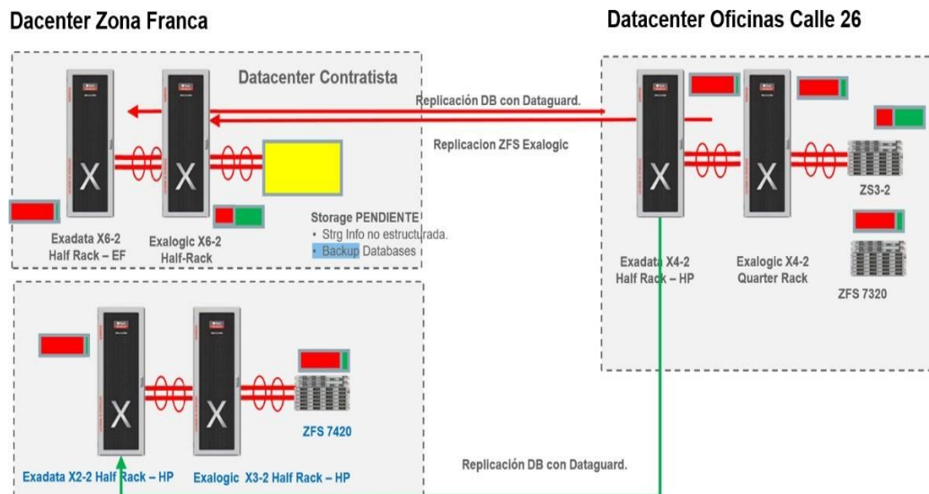
Figura 2. Infraestructura actual de Datacenter con equipo ORACLE
