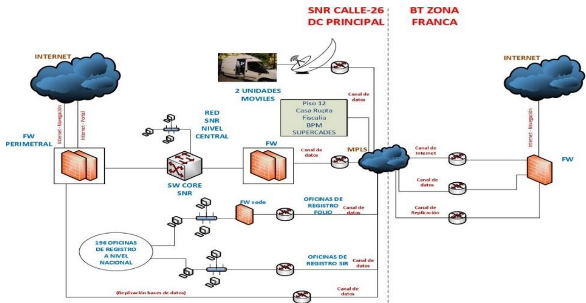
Figura 1. Infraestructura de comunicación SNR
