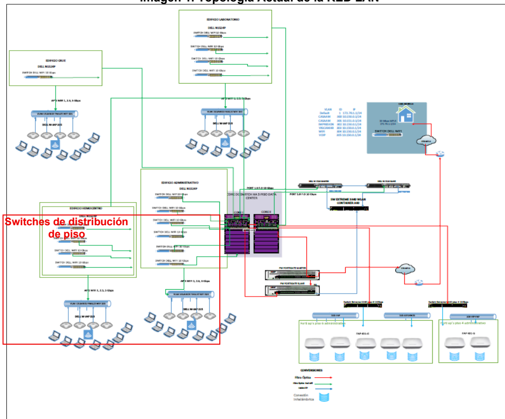
Imagen 1. Topología Actual de la RED LAN
