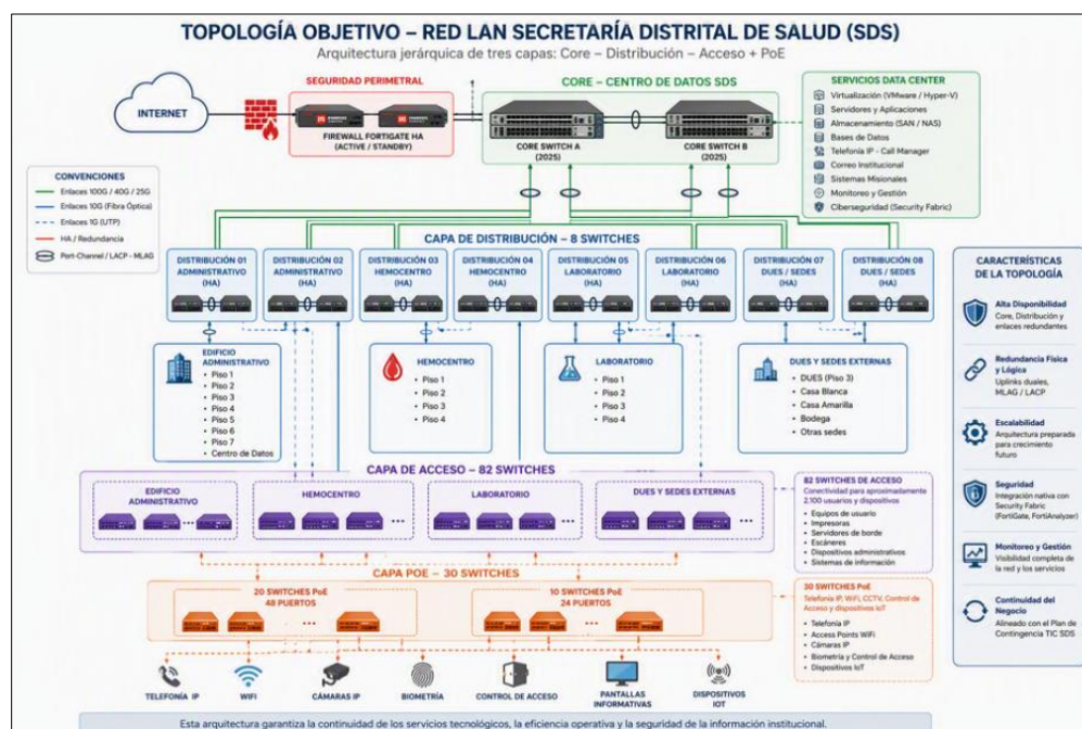
Imagen 4. Topología Objetivo de red LAN de la entidad con las nuevas conexiones de velocidad
