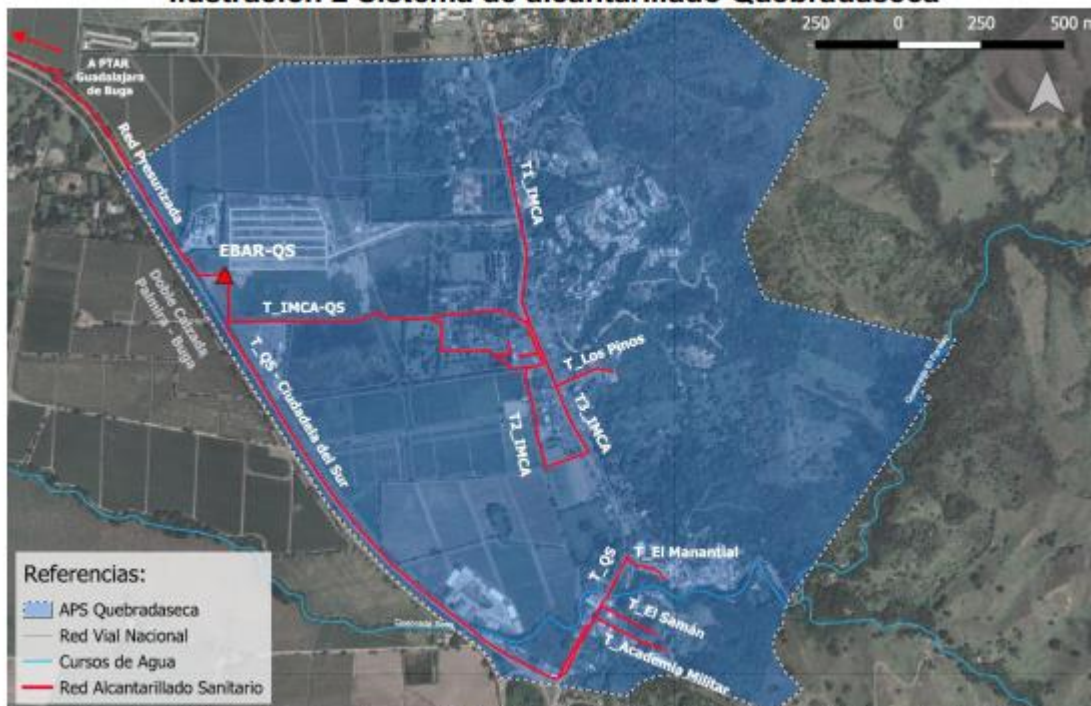
Ilustración 2 Sistema de alcantarillado Quebradaseca
