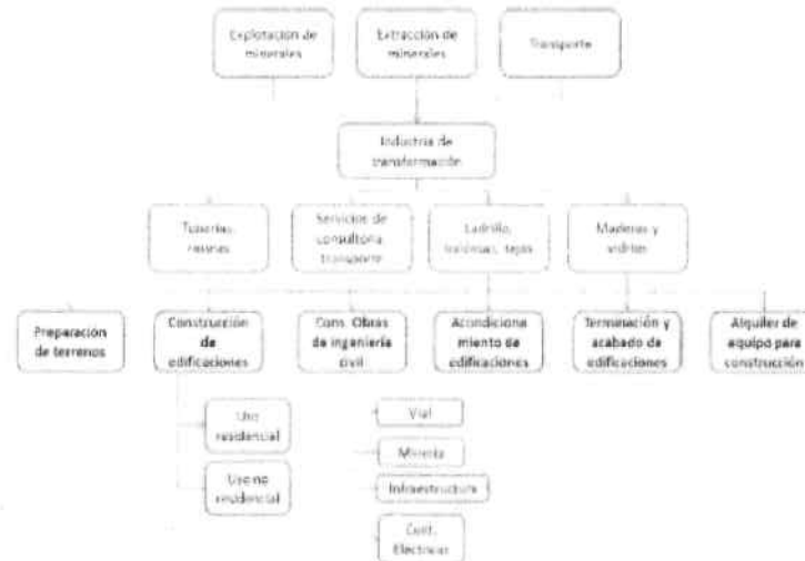
Gráfico 1. Cadena productiva
