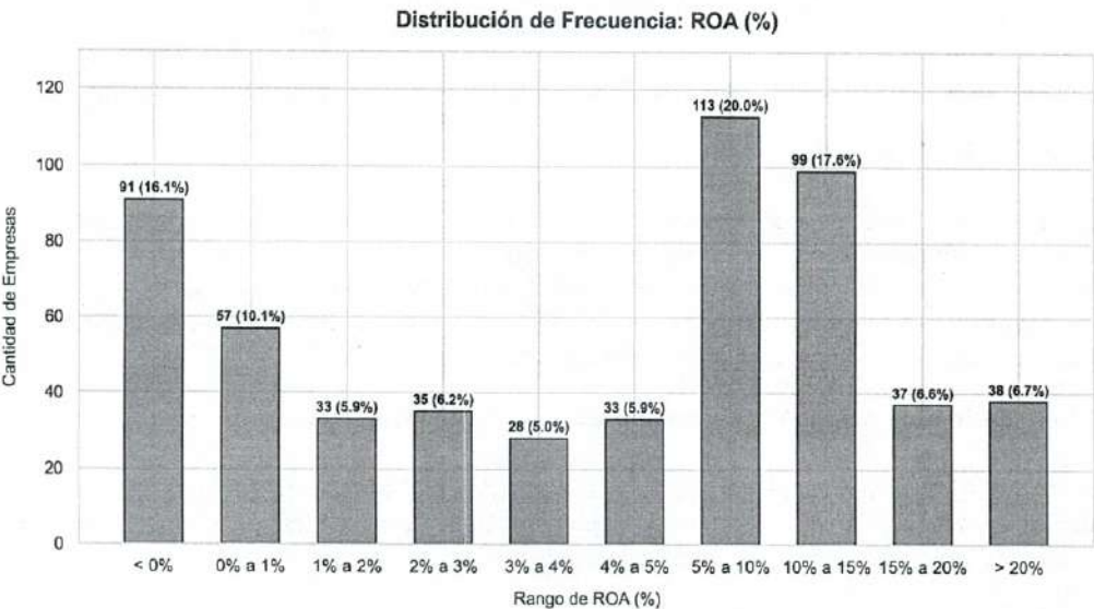
Ilustración 45. Distribución de frecuencia del Índice ROA sin outliers
