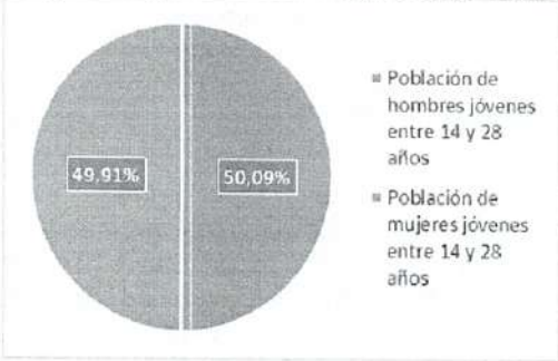
Ilustración 47. Proyección población de Ibagué entre 14 y 28 años - 2026
