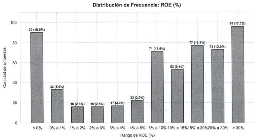
Ilustración 44. Distribución de frecuencia del Índice ROE sin outliers
