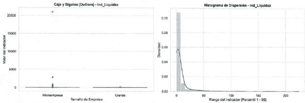
Ilustración 36. Diagrama de caja e histograma del Índice de liquidez con outliers
