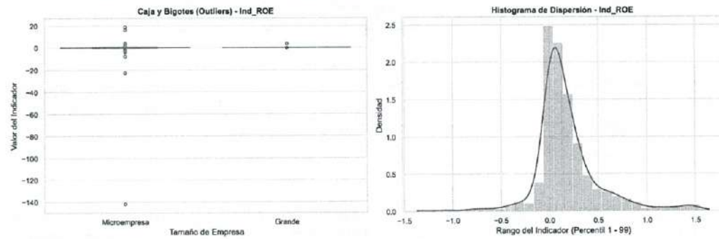
Ilustración 39. Diagrama de caja e histograma del Índice de ROE con outliers
