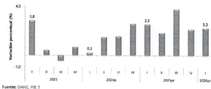
Ilustración 6. Producto Interno Bruto Tasa de crecimiento en volumen 2023-I / 2026 pr -I
