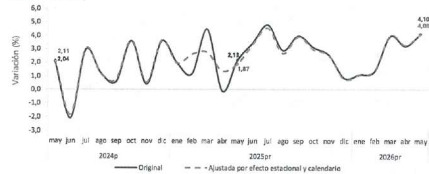
Ilustración 1. Tasa de crecimiento anual del índice del Indicador de Seguimiento a la Economía (ISE) Serie original y serie ajustada por efecto estacional y calendario 2024 p1 – 2026 pr2 (mayo)
