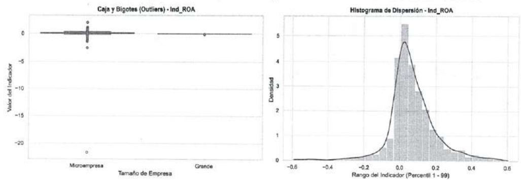
Ilustración 40. Diagrama de caja e histograma del Índice de ROA con outliers
