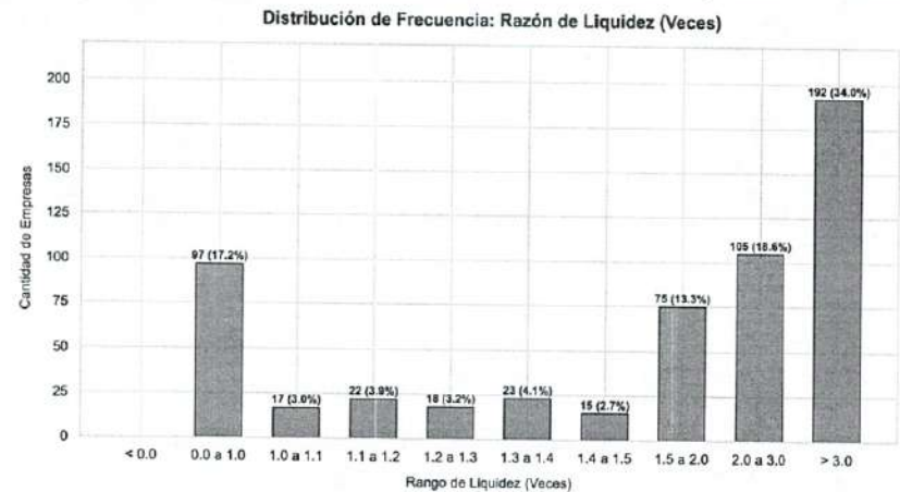
Ilustración 41. Distribución de frecuencia del Índice de Liquidez sin outliers
