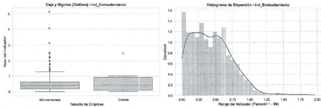
Ilustración 37. Diagrama de caja e histograma del Índice de endeudamiento con outliers
