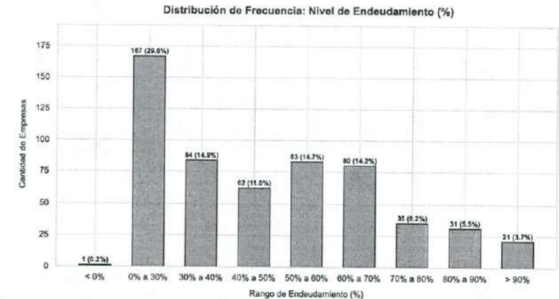
Ilustración 42. Distribución de frecuencia del Índice de endeudamiento sin outliers
