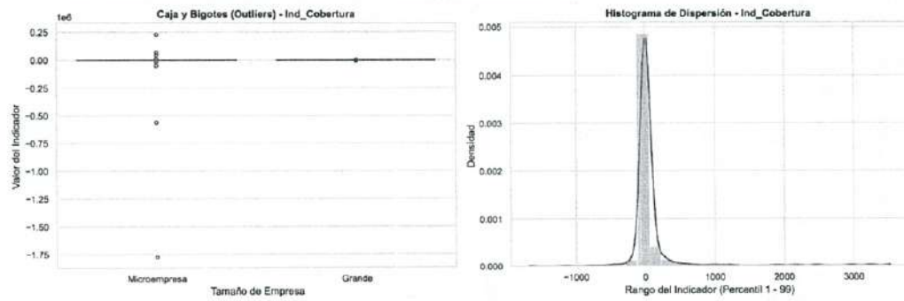
Ilustración 38. Diagrama de caja e histograma del Índice de cobertura con outliers
