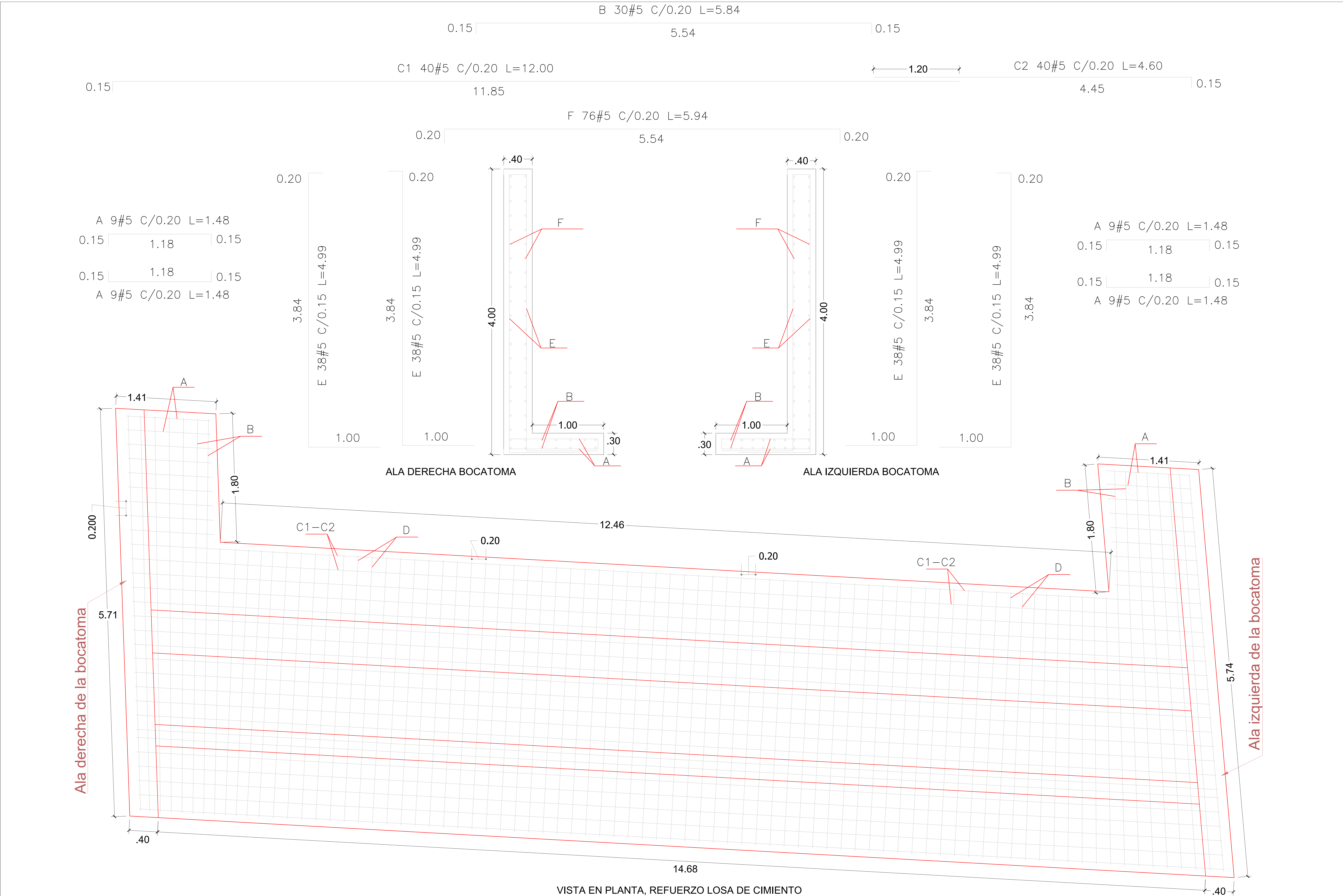
VISTA EN PLANTA, REFUERZO LOSA DE CIMENTO (ESTRUCTURA DE CAPTACIÓN-BOCATOMA)
