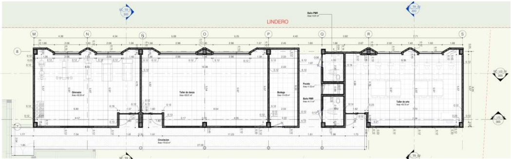
Imagen No. 4. Plano Planta Talleres
