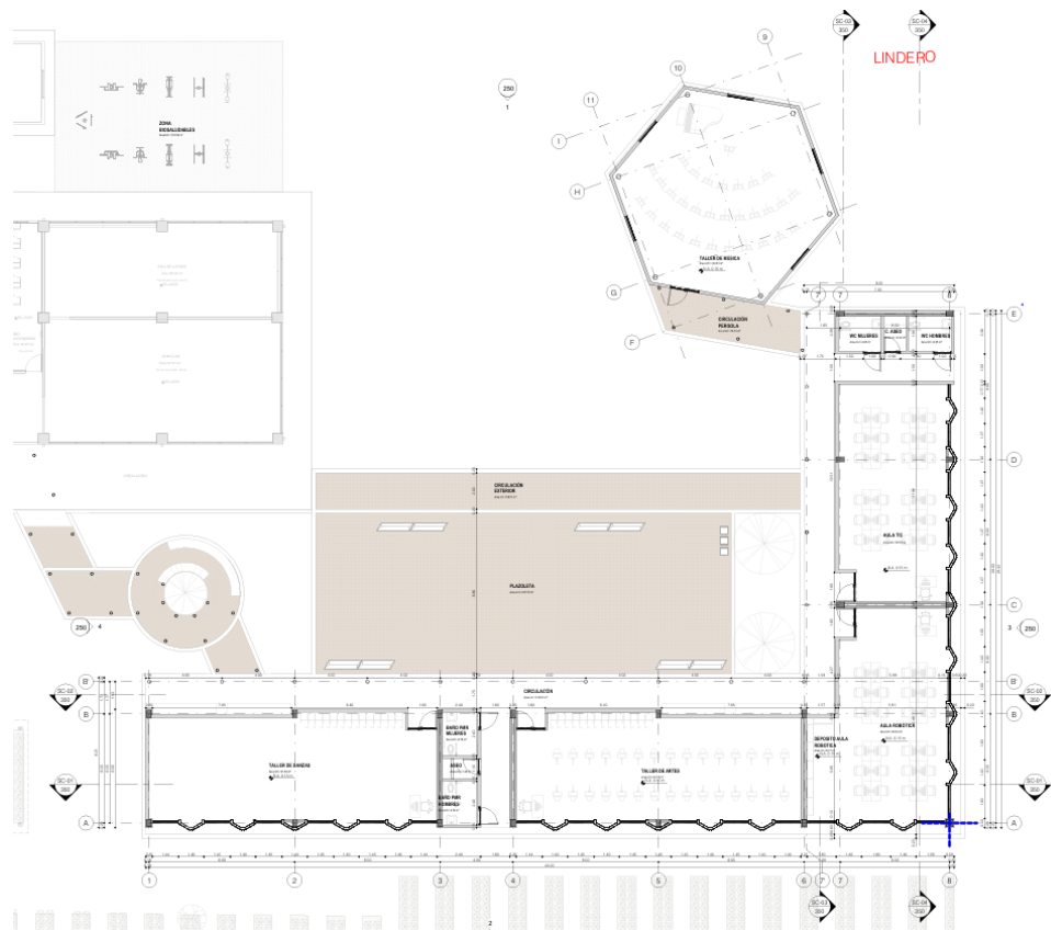
Imagen No. 4. Plano Planta Primer Piso
