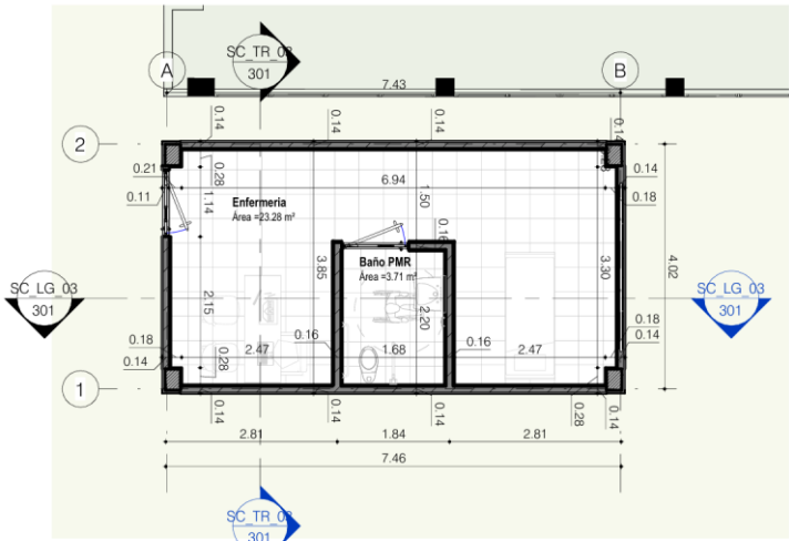
Imagen No. 6. Plano Planta Enfermería
