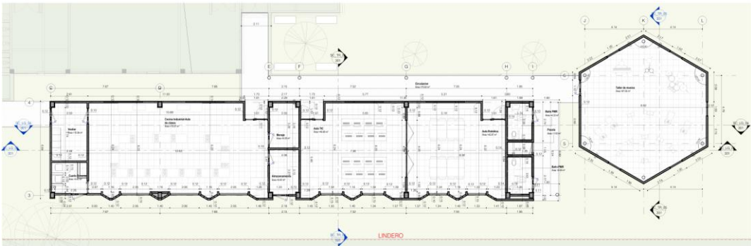
Imagen No. 5. Plano Planta Aulas
