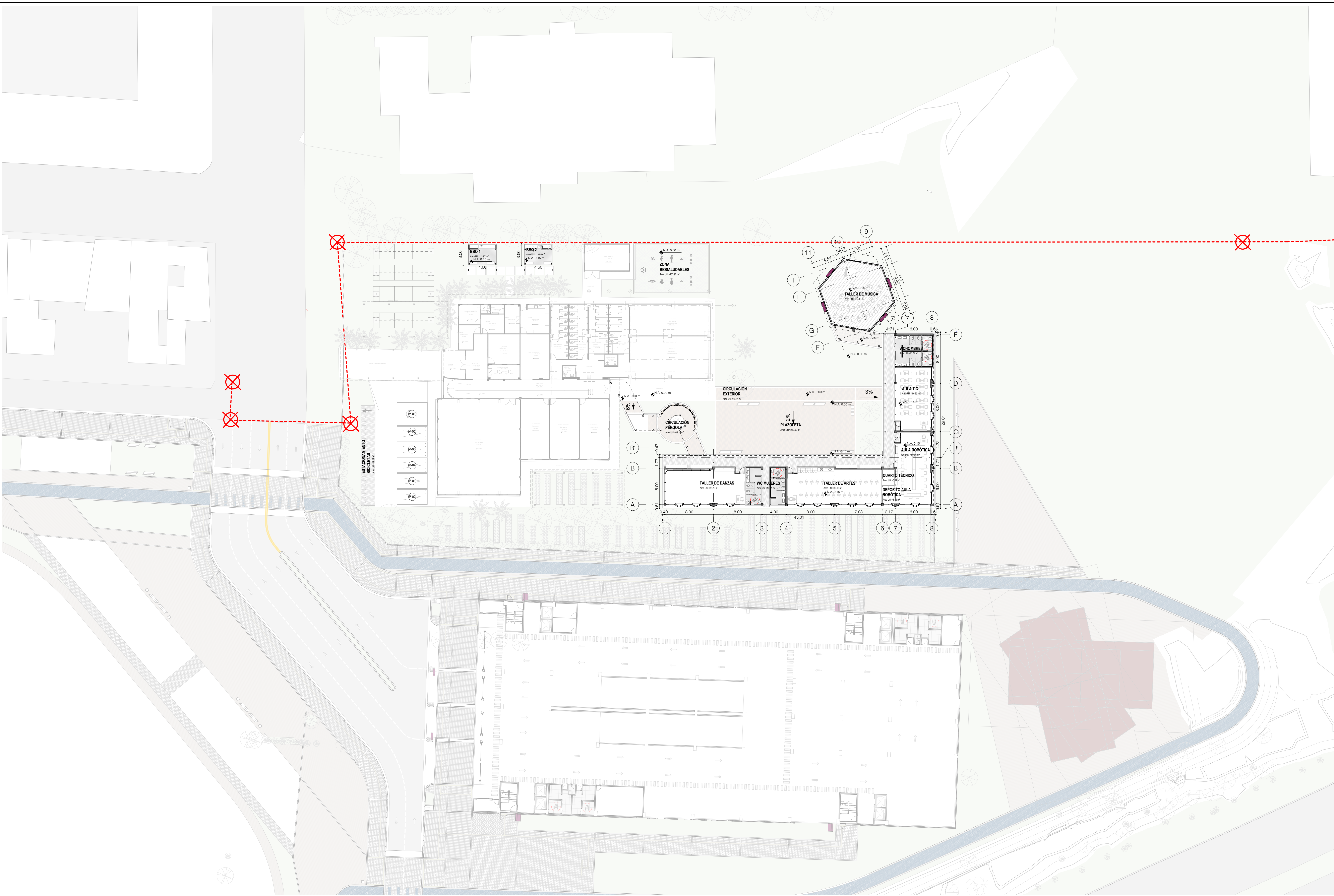
1 PLANTA IMPLANTACIÓN NIVEL L0 1 : 250
